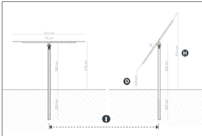
FIGURA 3: DEFINIZIONE DELLE DIMENSIONI DEI TRACKER
