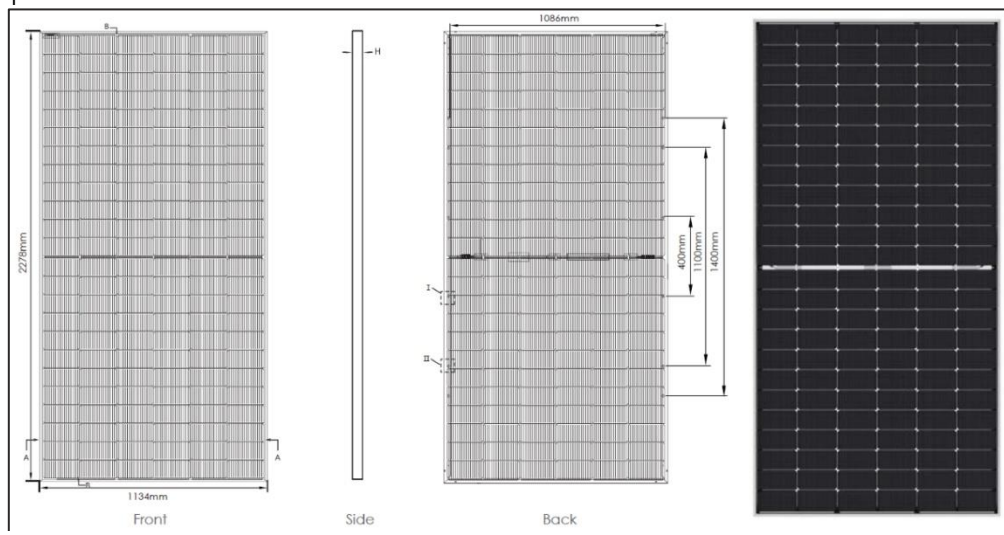
FIGURA 1 PANNELLO FV PARI A 570 WP – IN CONDIZIONI STANDARD - CON DIMENSIONI 2278 × 1134 × 35 MM
