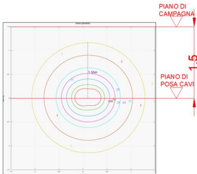
FIGURA 2: CURVE ISOINDUZIONE – 2 LINEE AT INTERRATE
