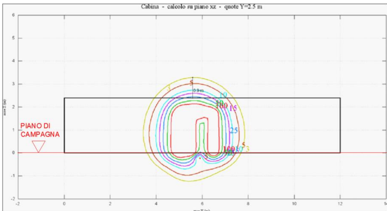
FIGURA 4: CURVE ISOINDUZIONE CABINA AT COLLETTORE (PROSPETTO FRONTALE)
