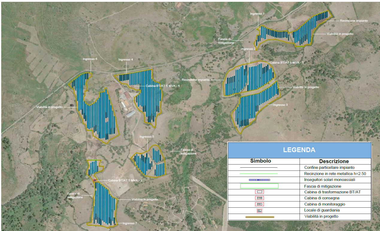
FIGURA 1 – LAYOUT PLANIMETRICO DELL’AREA D’IMPIANTO – LOTTO A NORD
