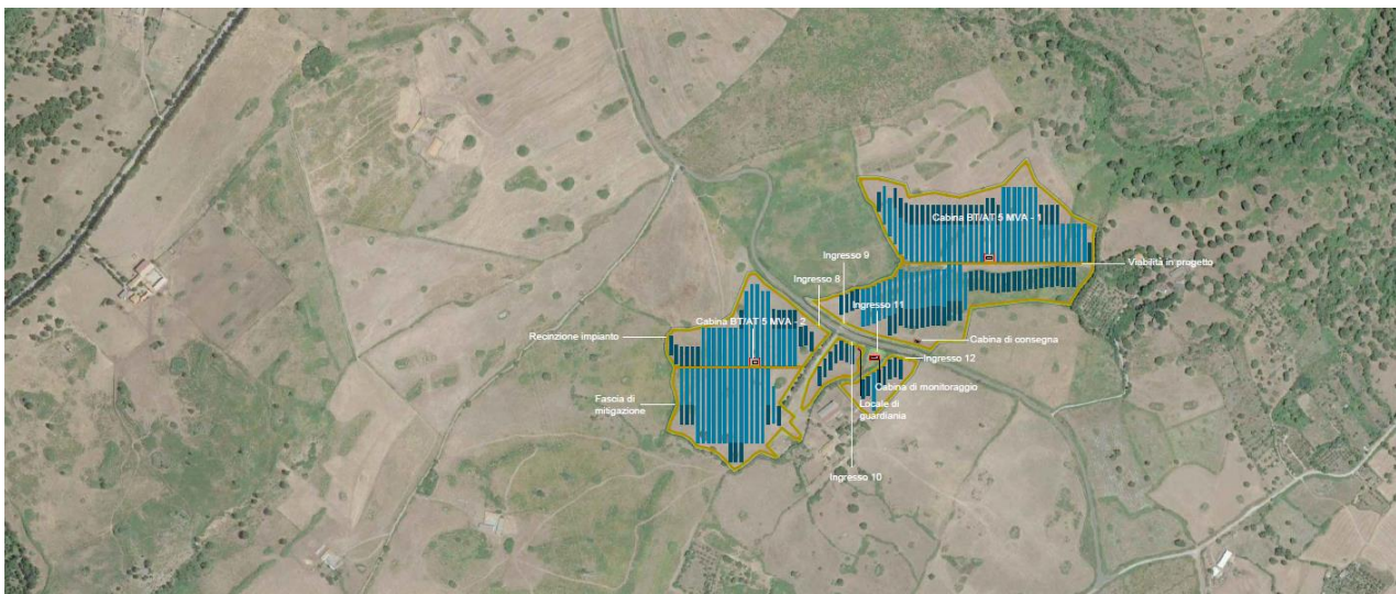
FIGURA 2 - LAYOUT PLANIMETRICO DELL’AREA D’IMPIANTO – LOTTO A SUD
