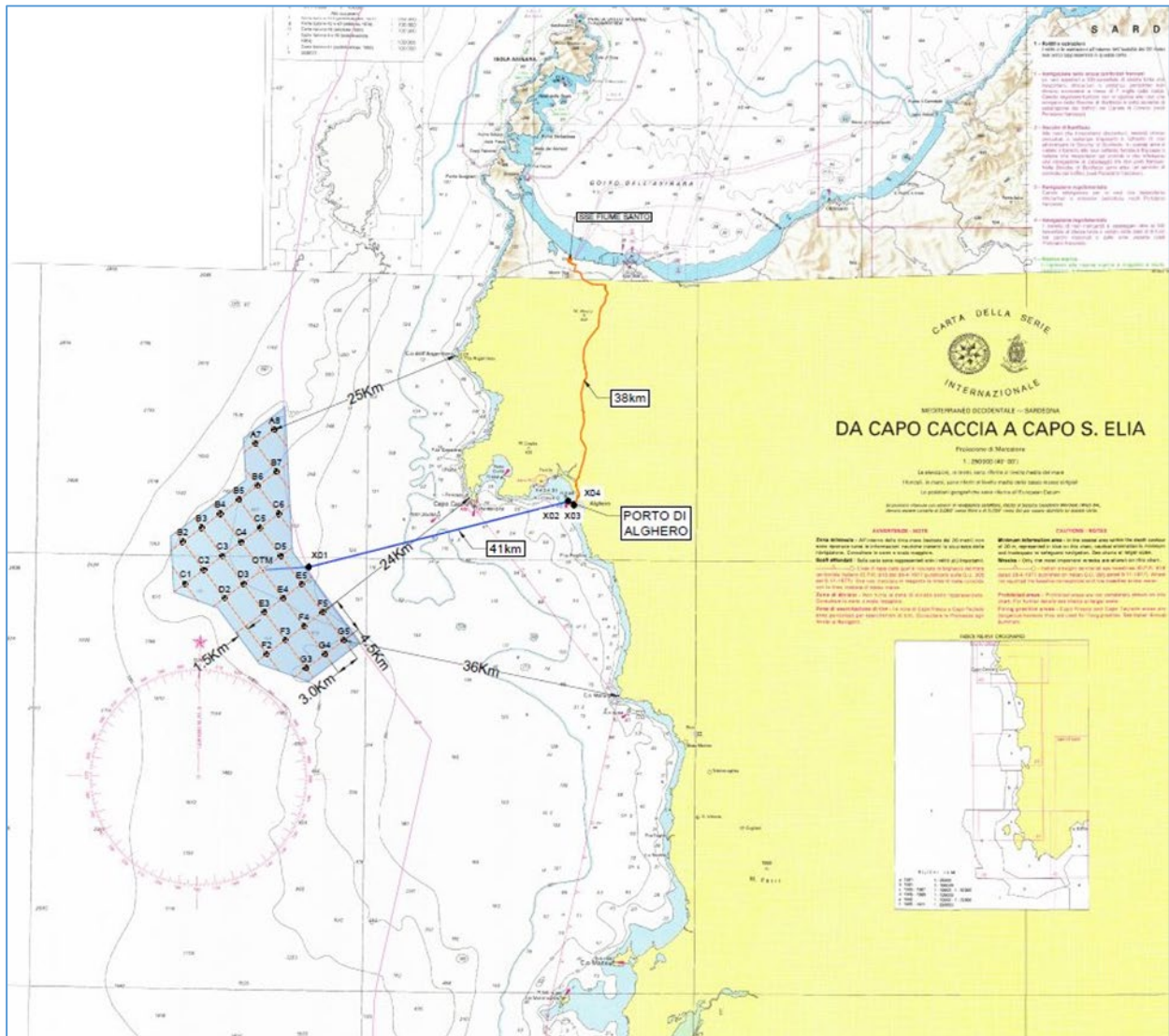
Figura 2: Layout impianto su carta nautica di dettaglio
