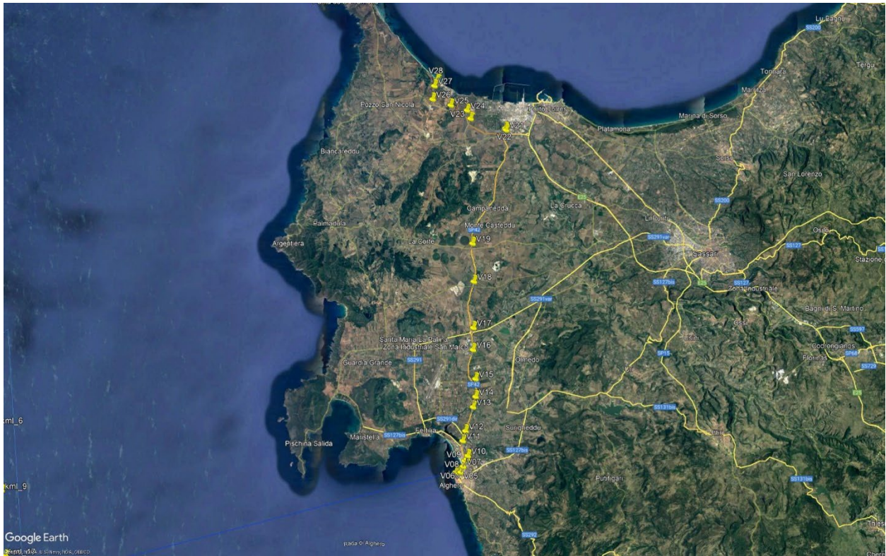
Percorso del cavidotto a terra dal punto di sbarco sul molo di ponente del Porto di Alghero, fino alla Stazione Elettrica di consegna di Terna "SE Fiume Santo".
