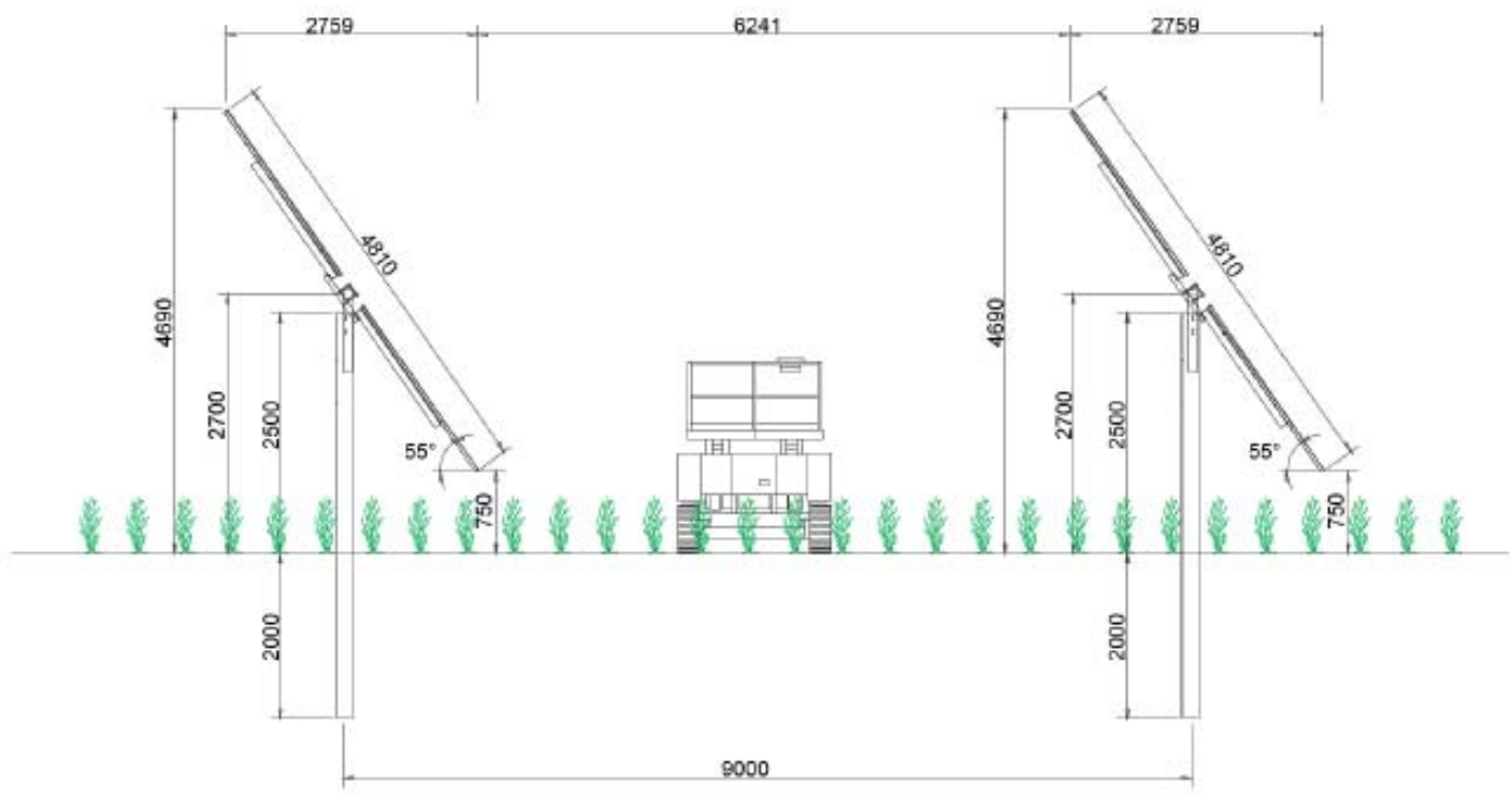
Figura 12 - Struttura di supporto con distanza tra i tracker.
