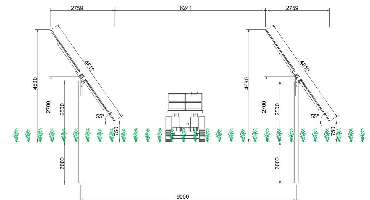
Tracker - Configurazione massima rotazione - Sezione laterale
