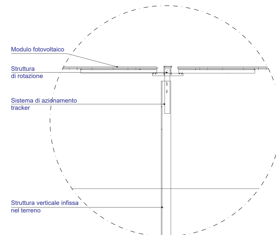
Tracker - Sezione di dettaglio
