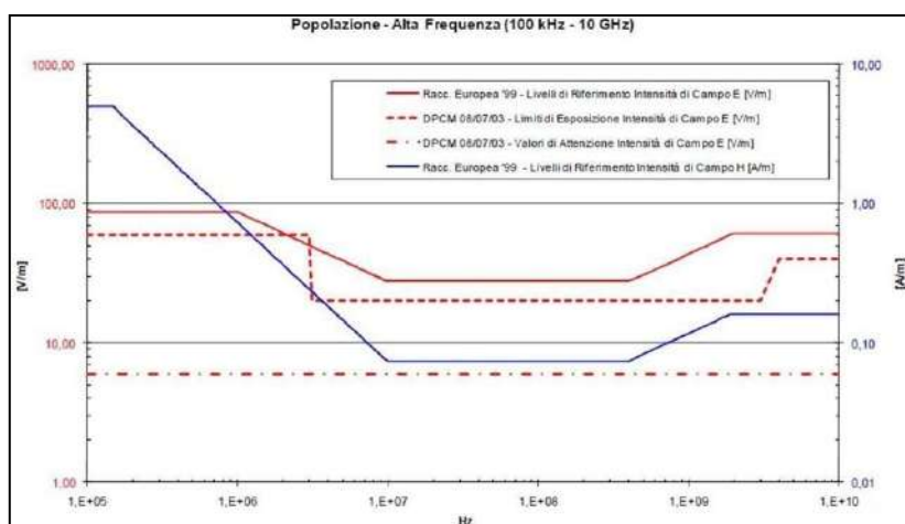
Figura 13.8. – Livelli esposizione Alta Frequenza (100kHz – 10 GHz).
