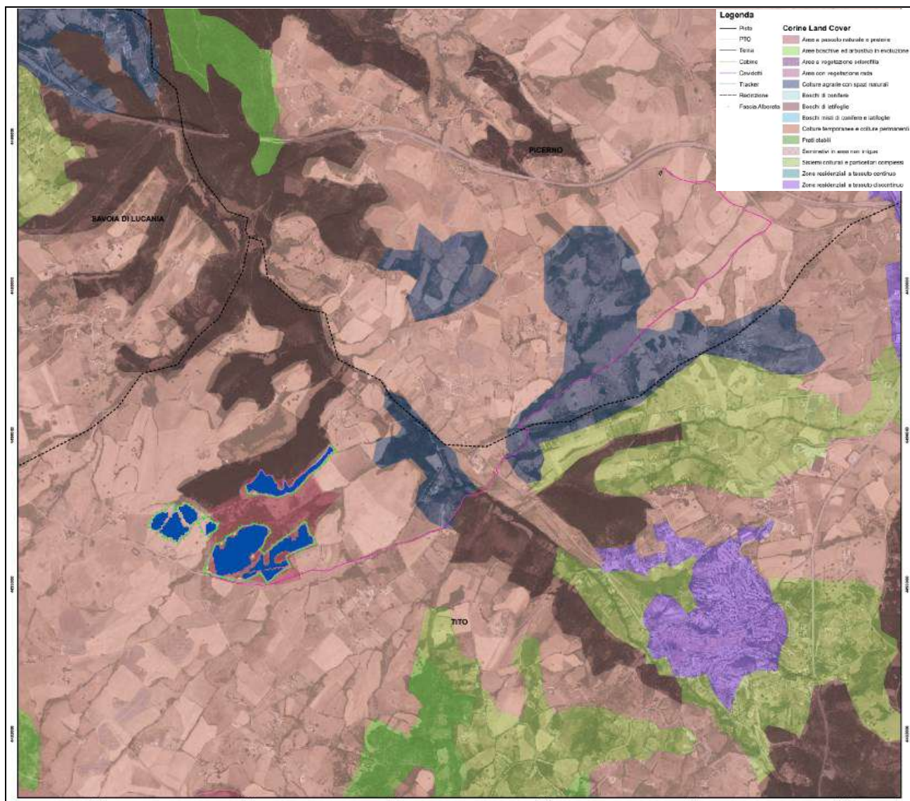
Figura 13.2. – Carta Uso del Suolo Corine Land Cover.
