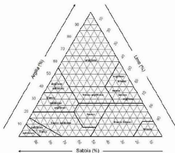
Figura 13.4. – Classificazione Tessiturale del terreno USDA.
