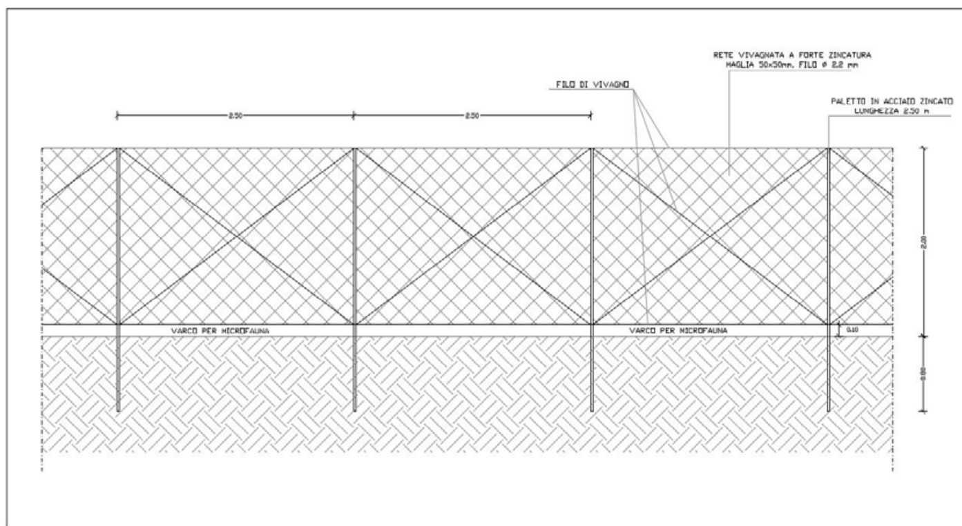
Recinzione tipo dell'Area del Campo Agrivoltaico
