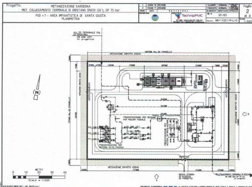
(da ENURA S.p.A. – Metanizzazione Sardegna – Tratto Sud, elaborato n. ST-153, Foglio 2 di 3)
