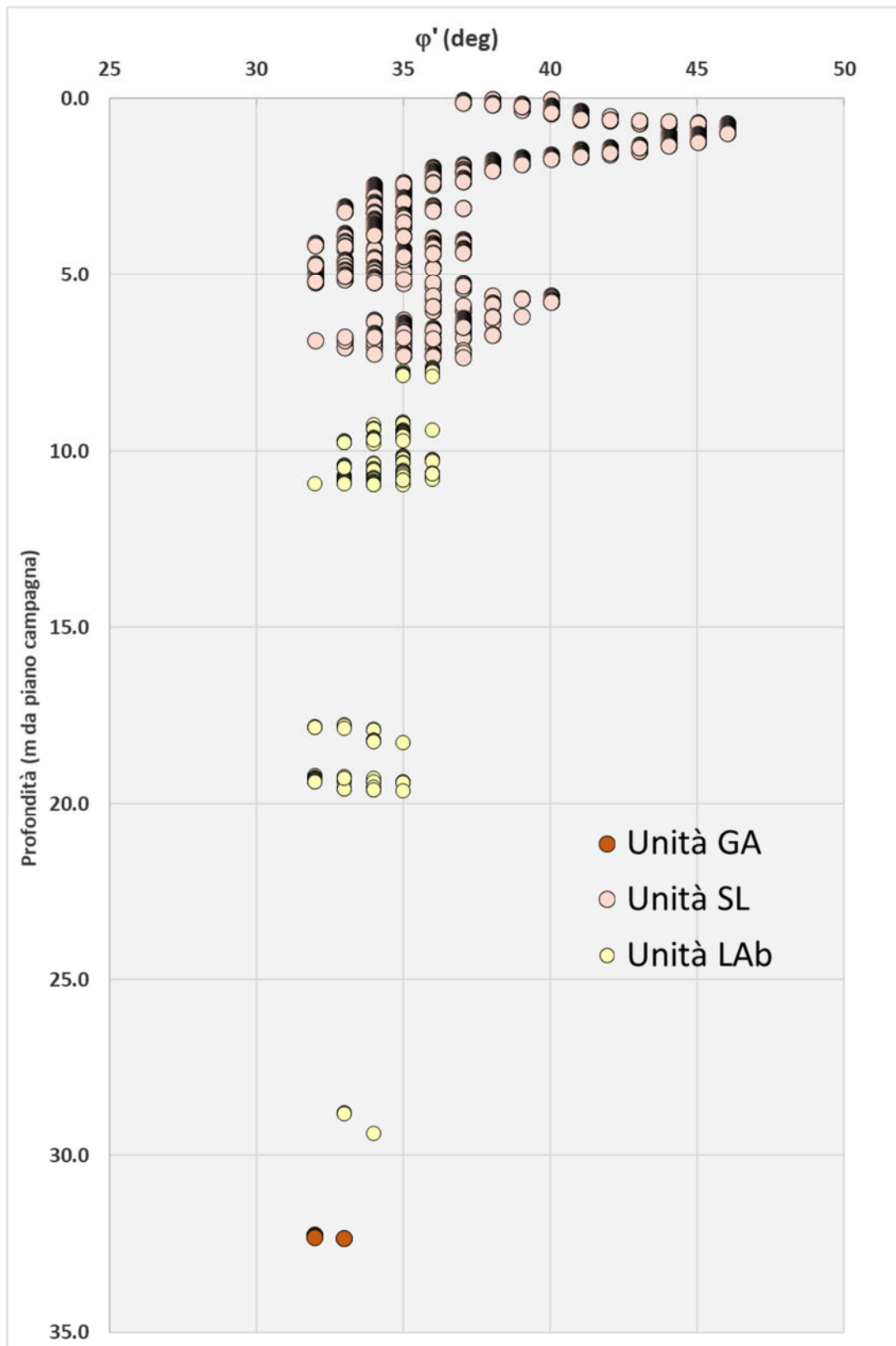
Figura 3 Profilo angolo di attrito unità incoerenti
