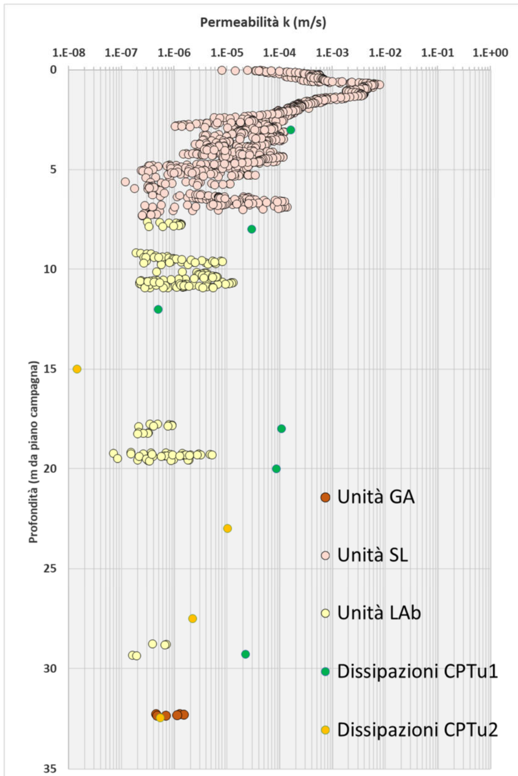
Figura 5 Profilo permeabilità unità incoerenti
