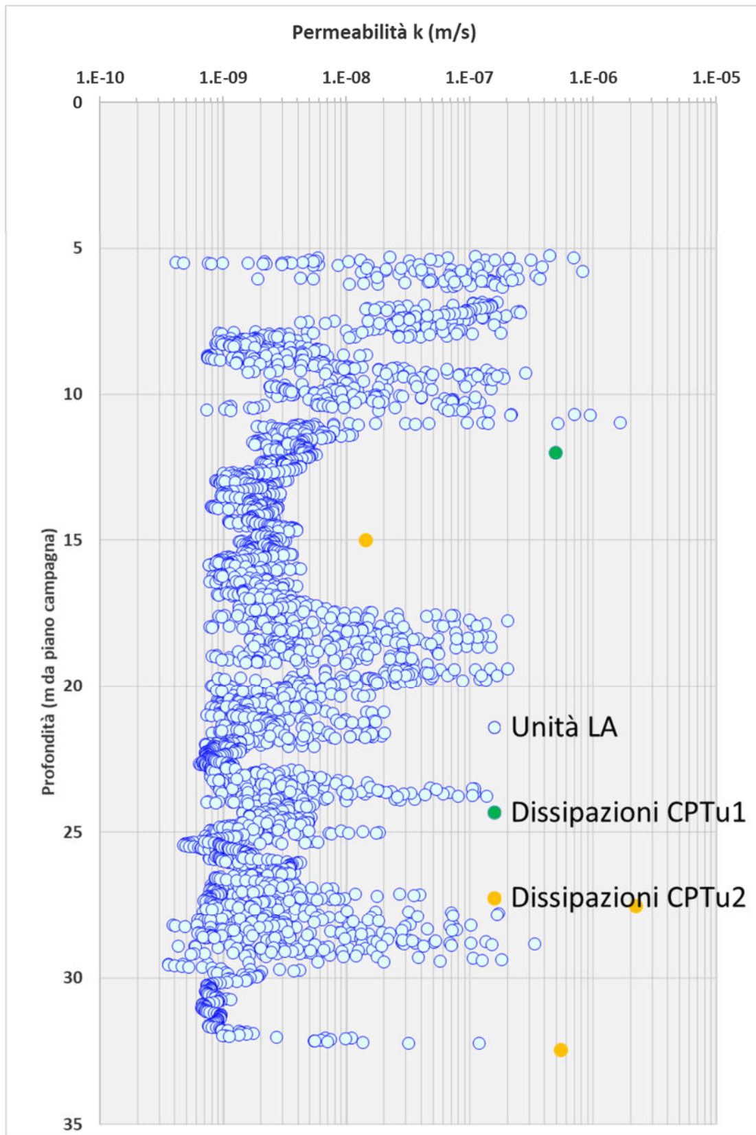
Figura 11 Profilo permeabilità unità coesive
