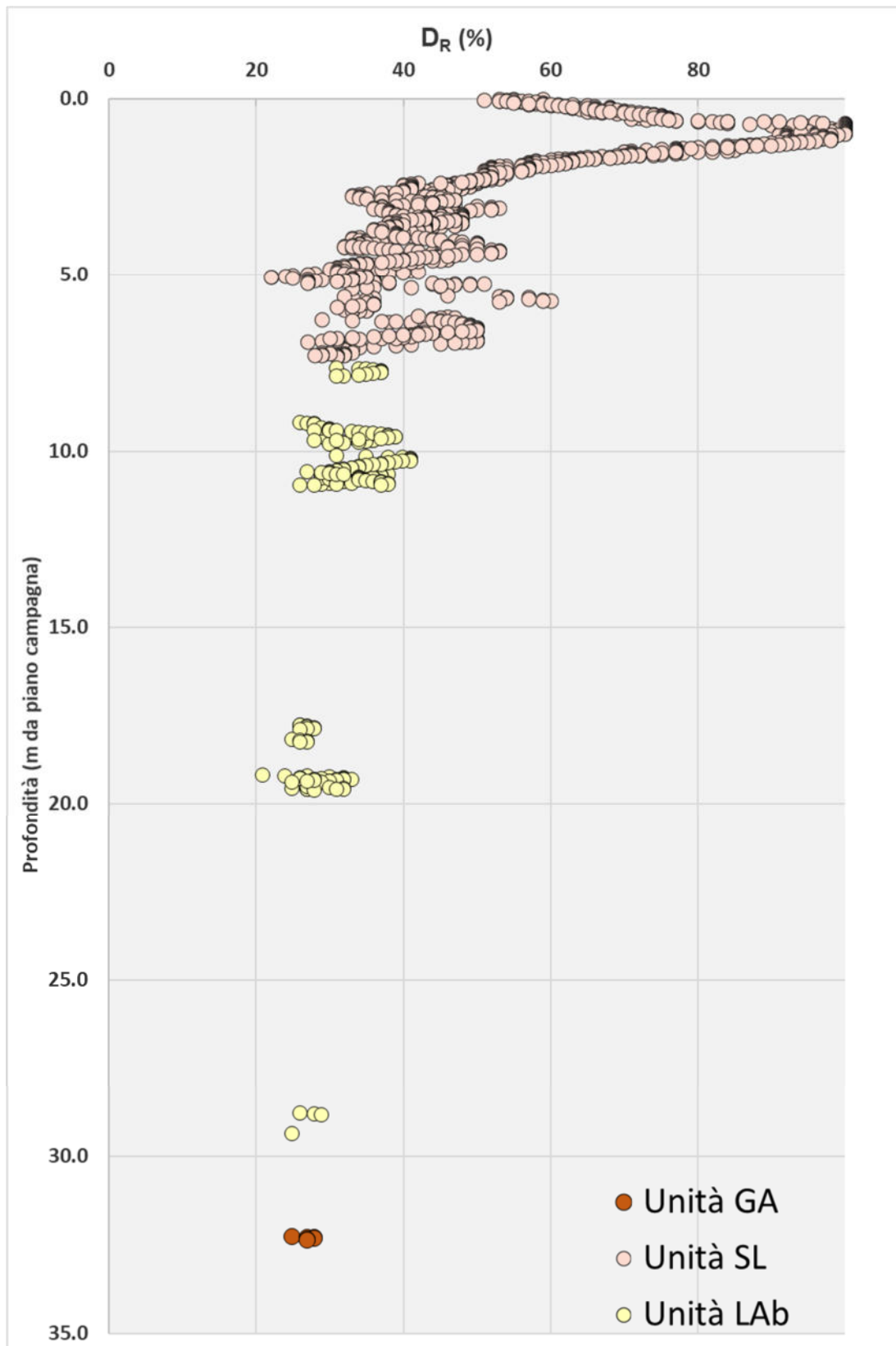
Figura 2 Profilo densità relativa unità incoerenti
