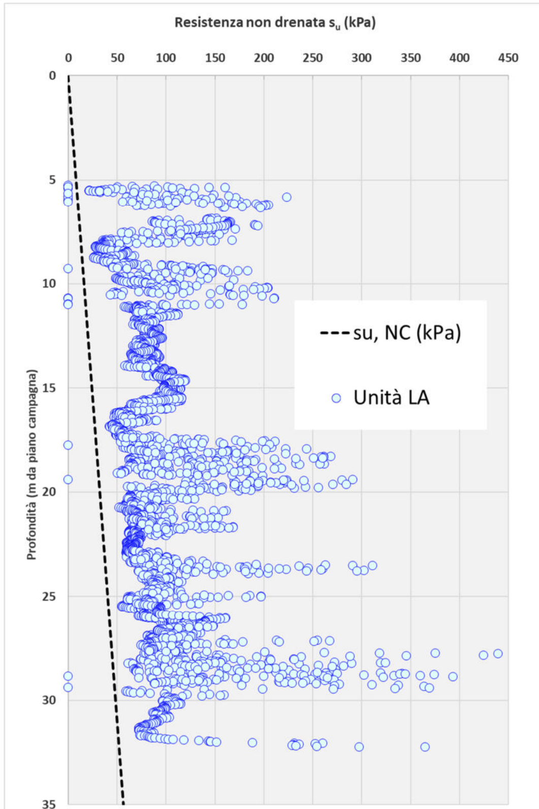
Figura 7 Profilo resistenza non drenata unità coesive
