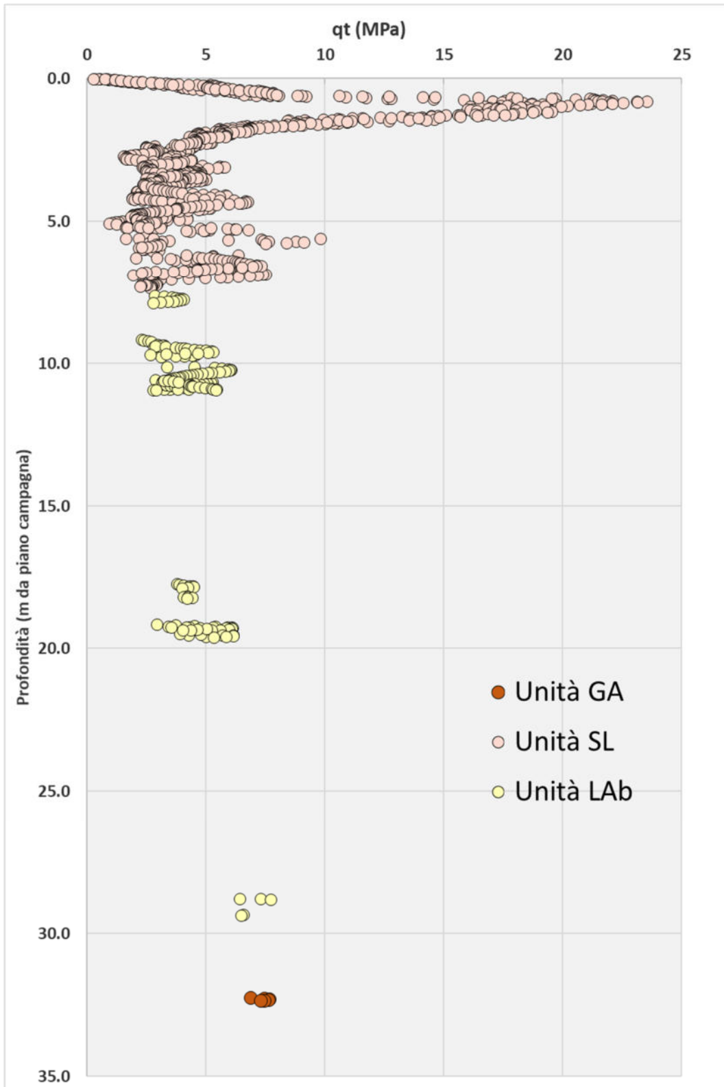
Figura 1 Profilo resistenza di punta unità incoerenti
