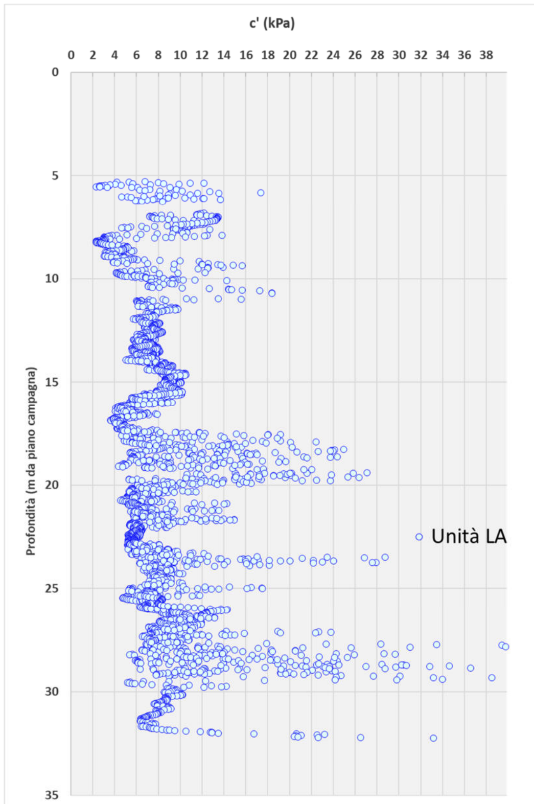
Figura 9 Profilo coesione efficace unità coesive
