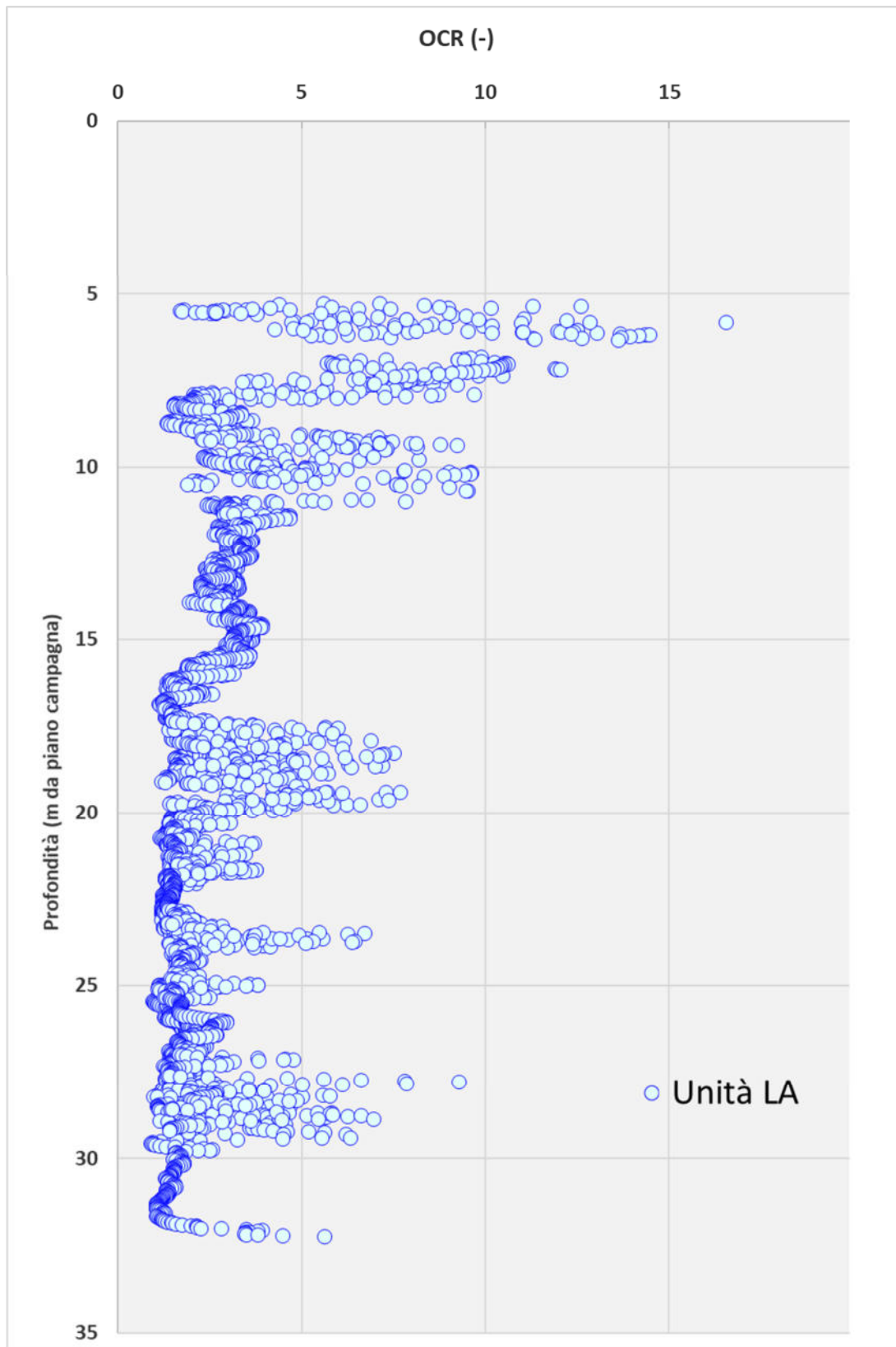
Figura 8 Profilo grado di sovraconsolidazione unità coesive
