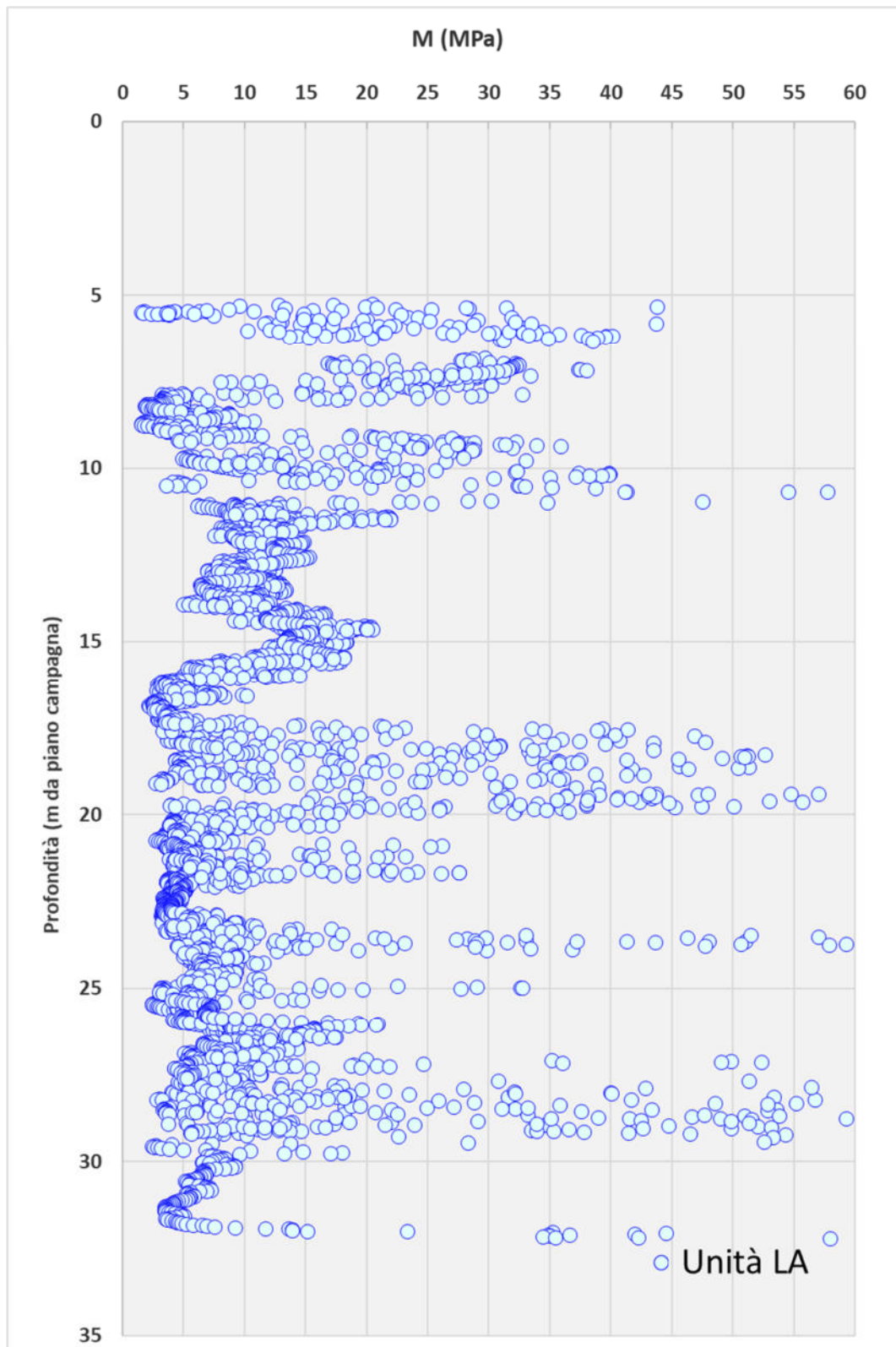
Figura 10 Profilo modulo edometrico unità coesive
