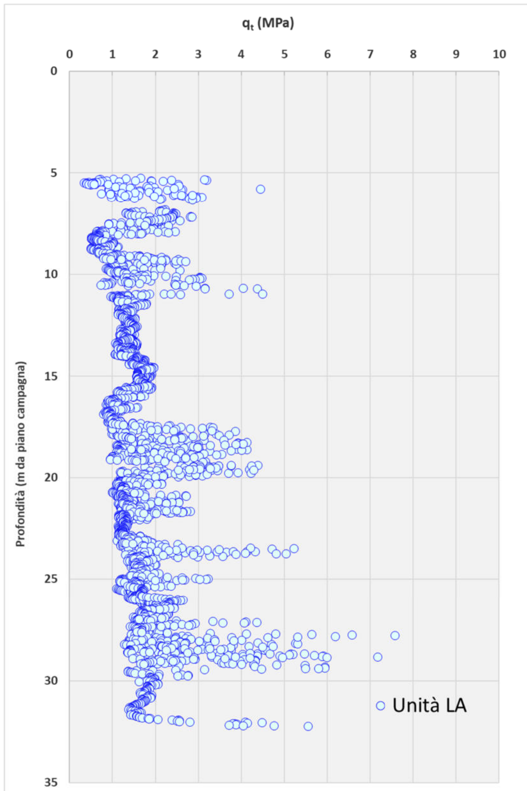
Figura 6 Profilo resistenza di punta unità coesive
