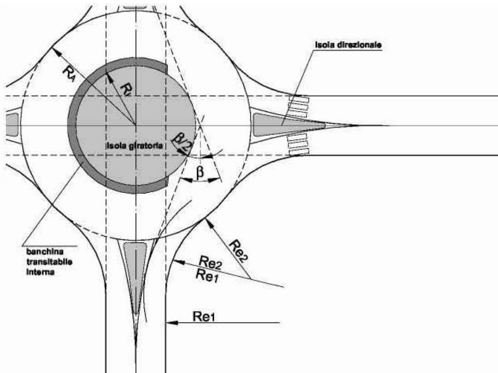
Fig 6.2 - Stralcio tipologico rotatoria
