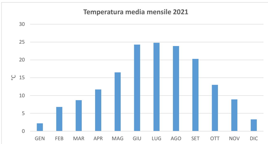
Figura 6 Temperatura media mensile
