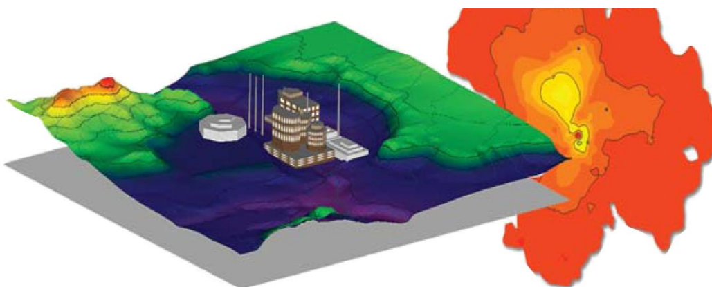
Figura 22 AermocView Esempio di modellazione grafica 3D delle curve di isoconcentrazione
