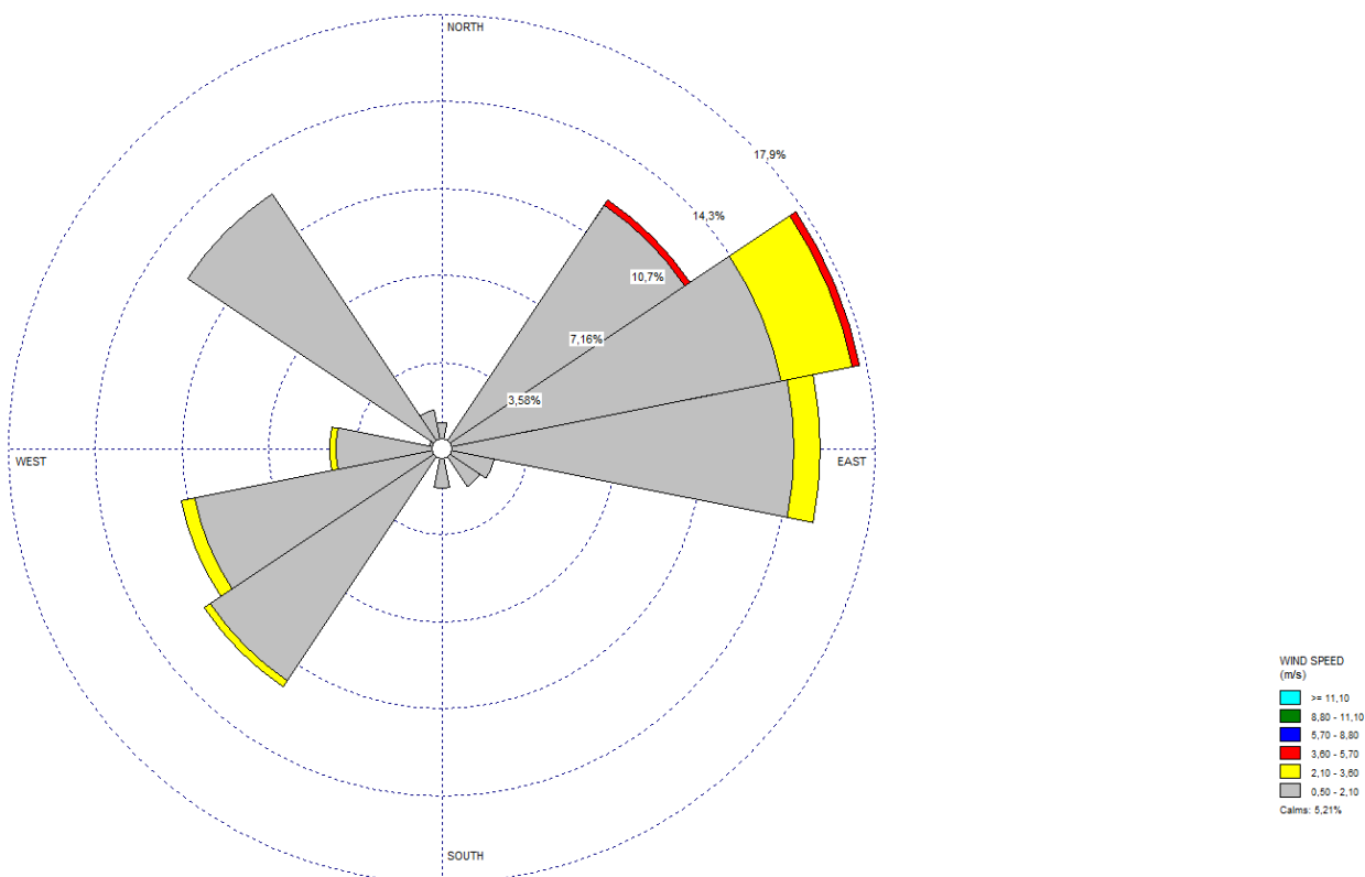
Figura 10 Rosa dei venti
