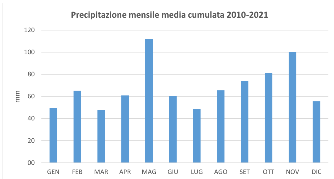
Figura 2 Precipitazione cumulativa media mensile
