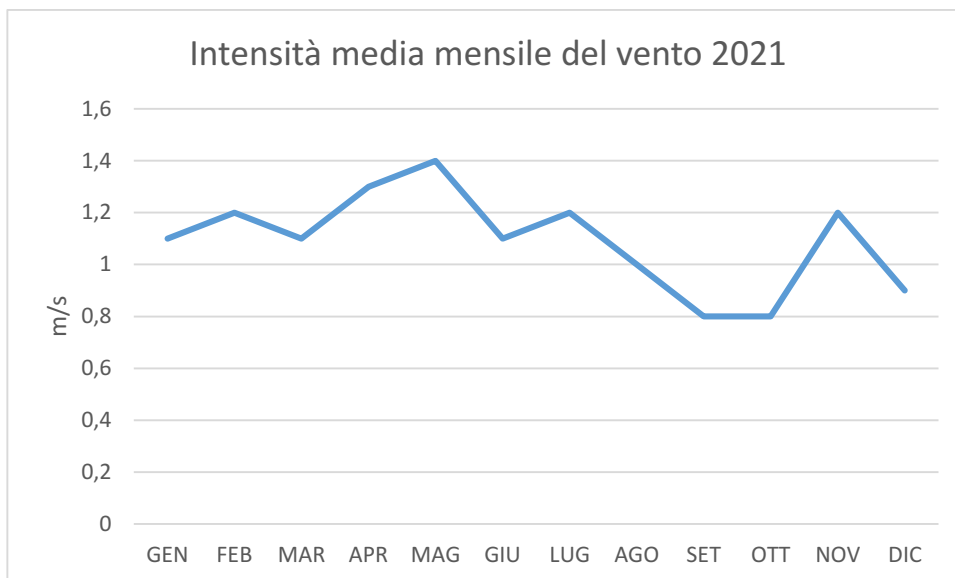
Figura 9 Velocità media del vento
