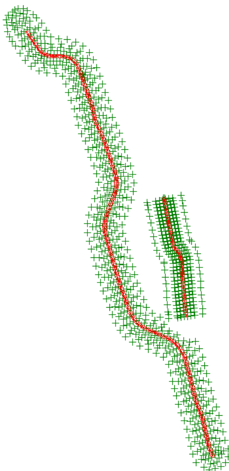
Figura 33 Rappresentazione grafica maglia di punti
