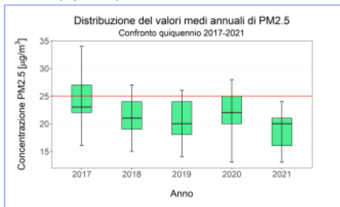
Figura 19 Distribuzione delle concentrazioni medie annue di particolato PM2.5. Confronto
