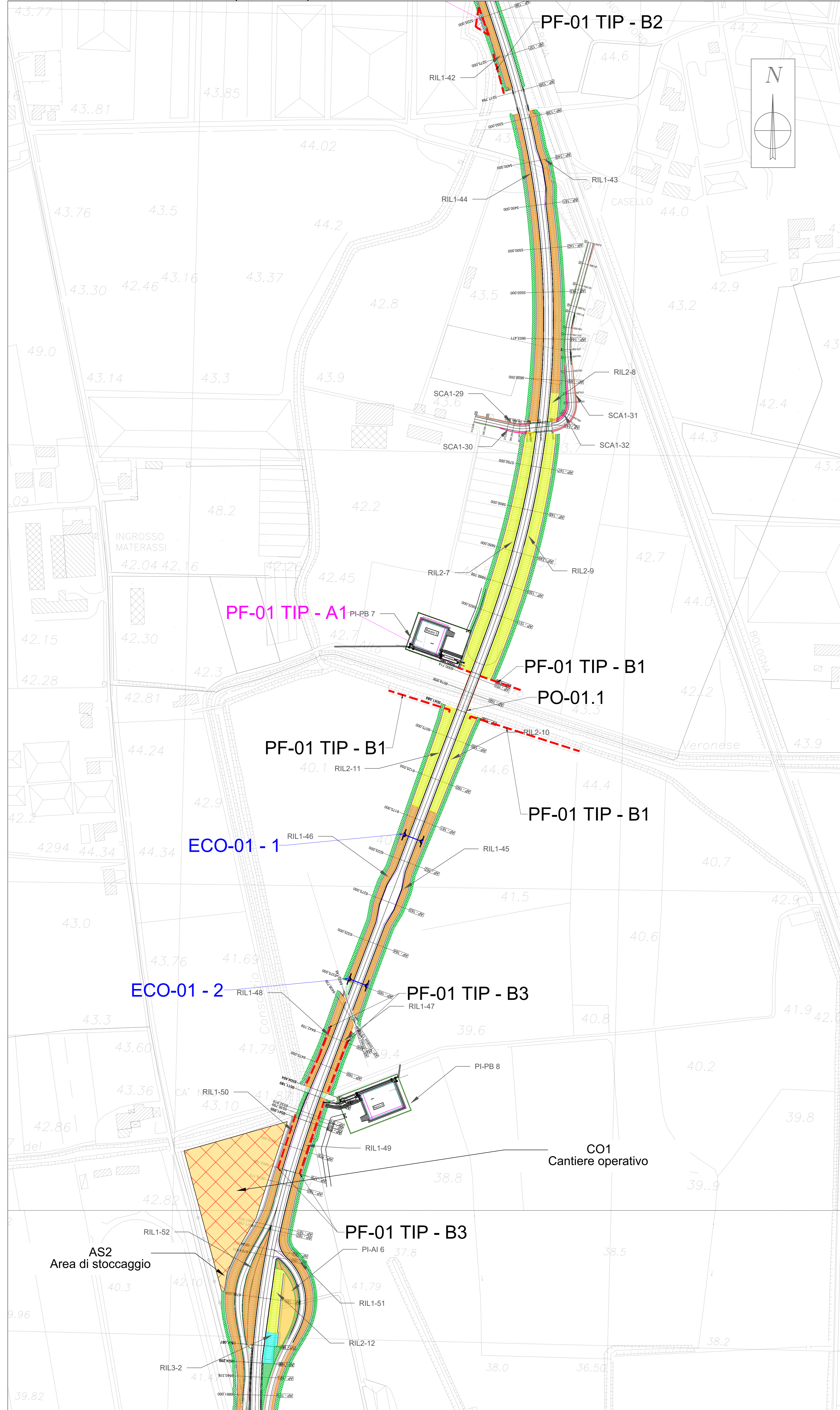
PLANIMETRIA OPERE A VERDE (Quadro 2c) - SC. 1:2.000
