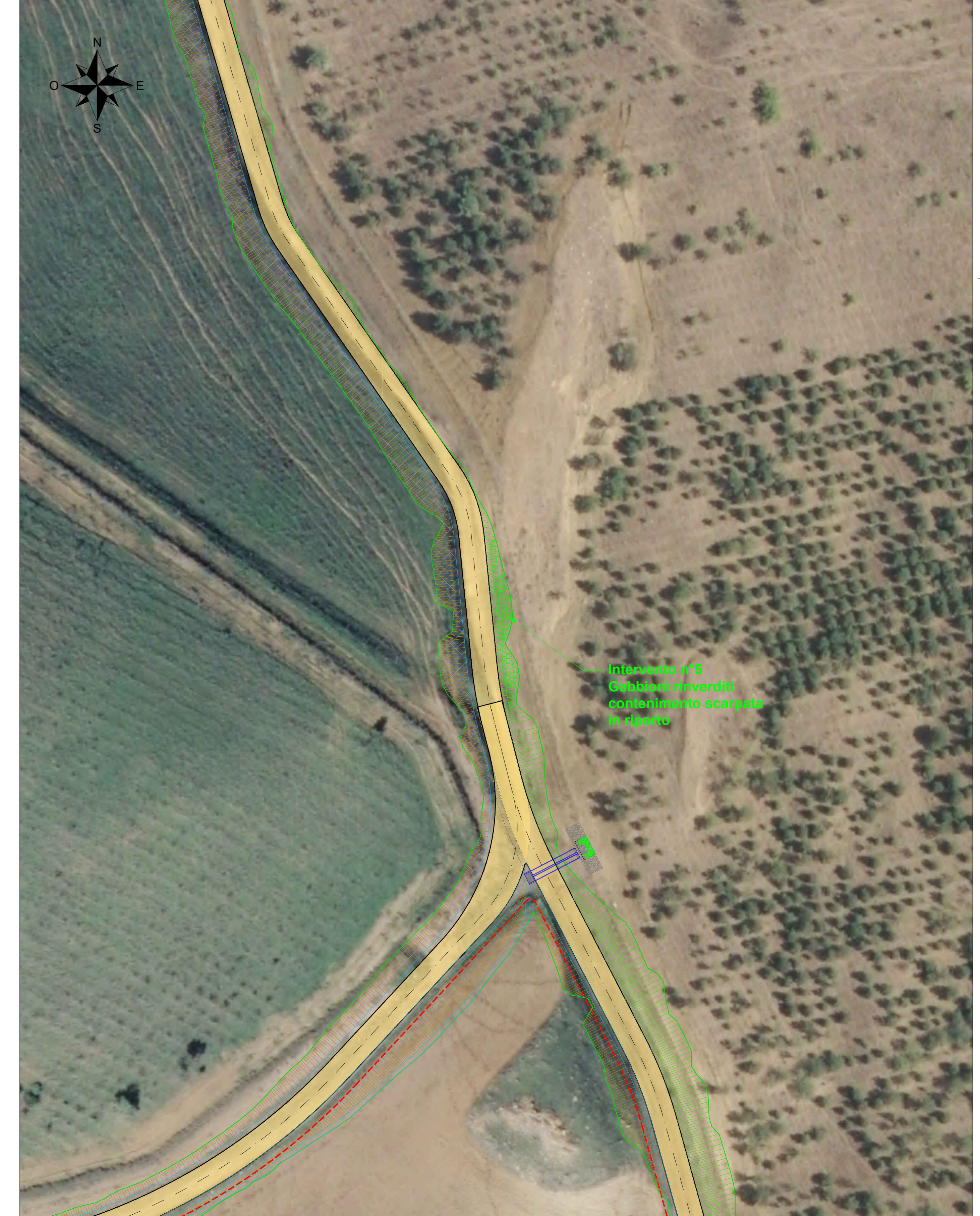
Intervento n°5 - Gabbioni rinverdit - Scala 1:500
