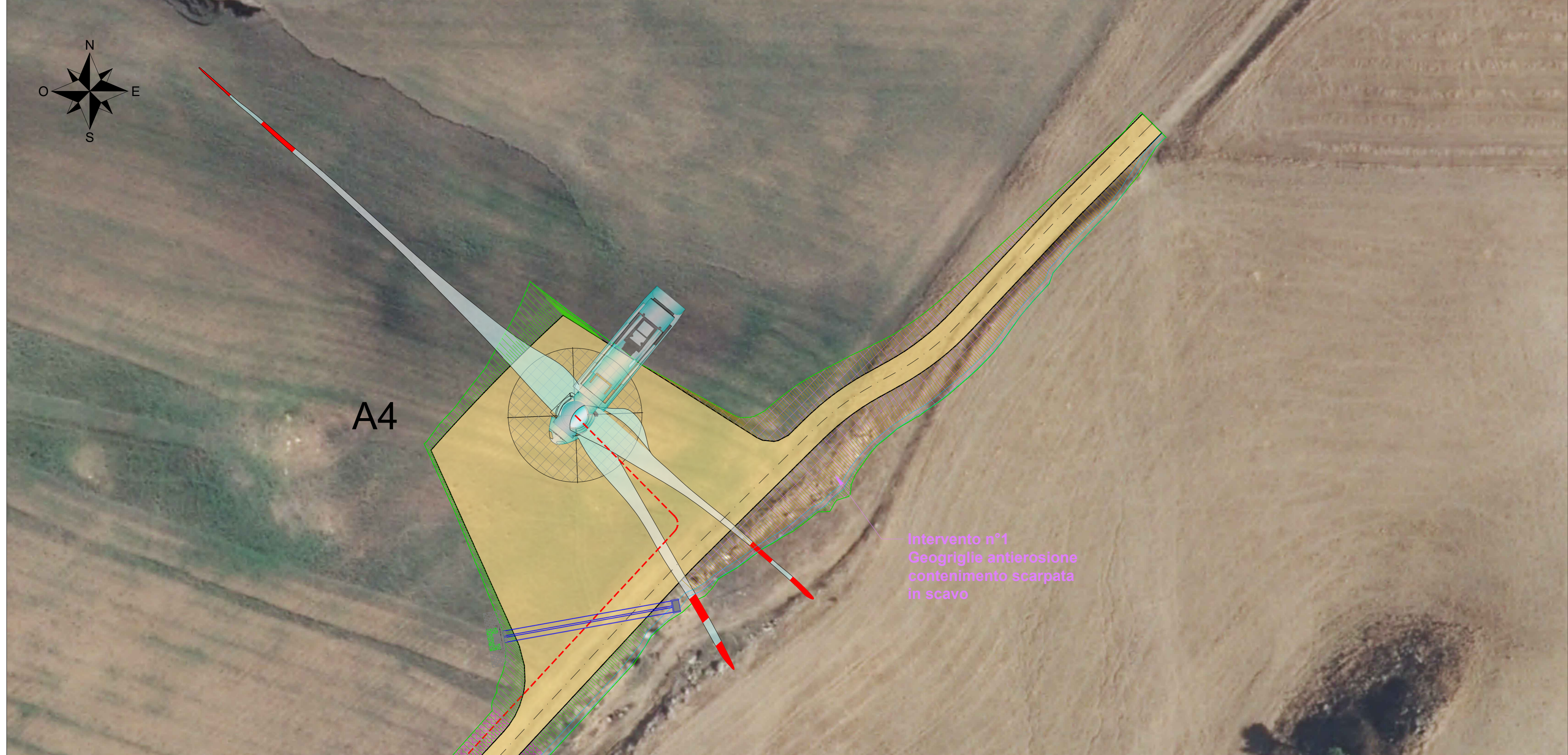
Intervento n°3 - Geogriglie antierosione - Scala 1:500
