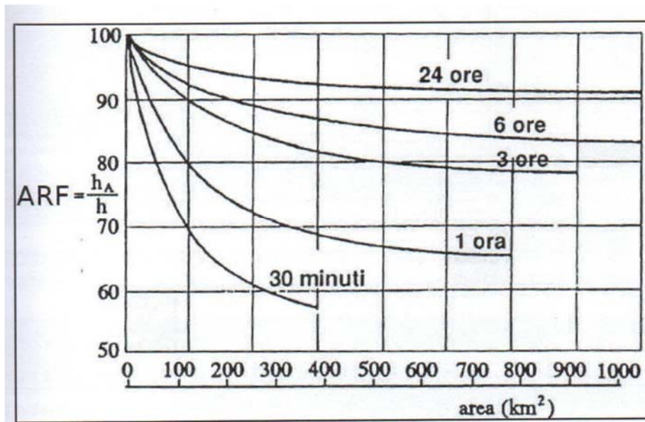
Fig. 5: Carta valutazione del coefficiente di riduzione areale
