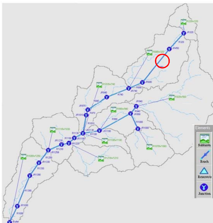
Fig. 11: Sottobacini idrografici del Fiume Belice con indicazione dell'area di interesse (da Relazione P.A.I. Bacino Fiume Belice- n. 057)
