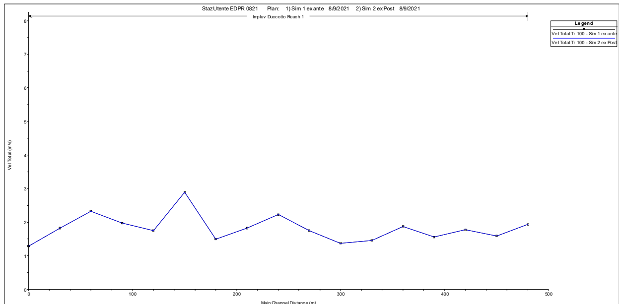
Fig. 15: Confronto longitudinale velocità flusso, ex ante / ex post; Tr 100 anni
