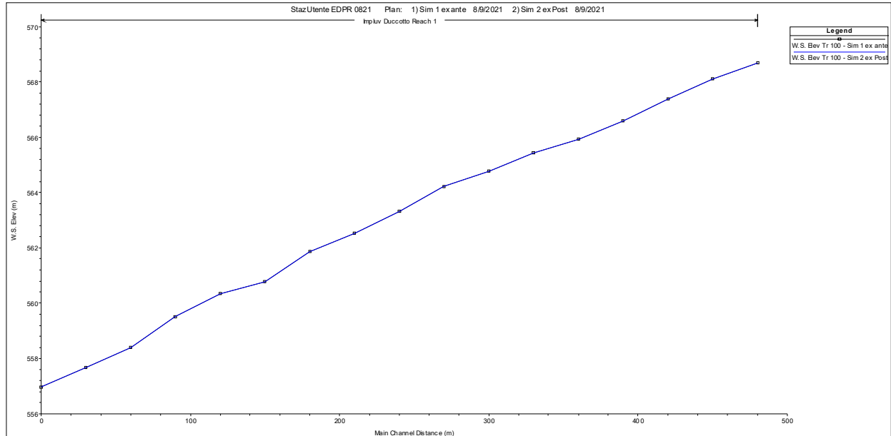
Fig. 14: Confronto longitudinale livello pelo Libero ex ante / ex post; Tr 100 anni
