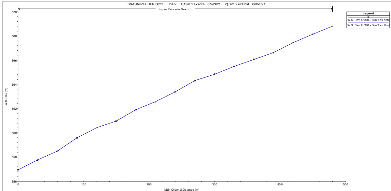
Fig. 17: Confronto longitudinale livello pelo Libero ex ante / ex post; Tr 300 anni
