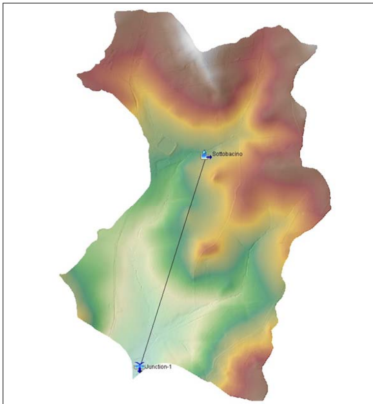
Fig. 8: Modellazione sottobacino in HEC-HMS
