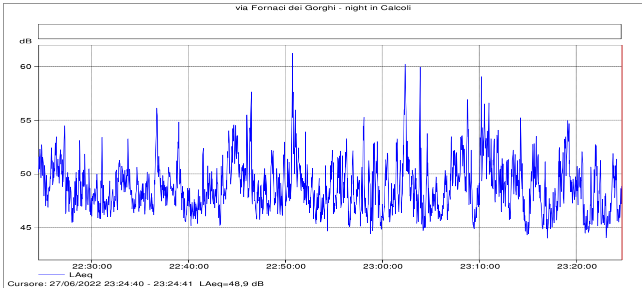
Fig.4.1.K- Centralina monitoraggio spot notturno – affaccio futura sottostazione – Time history livelli equivalenti
