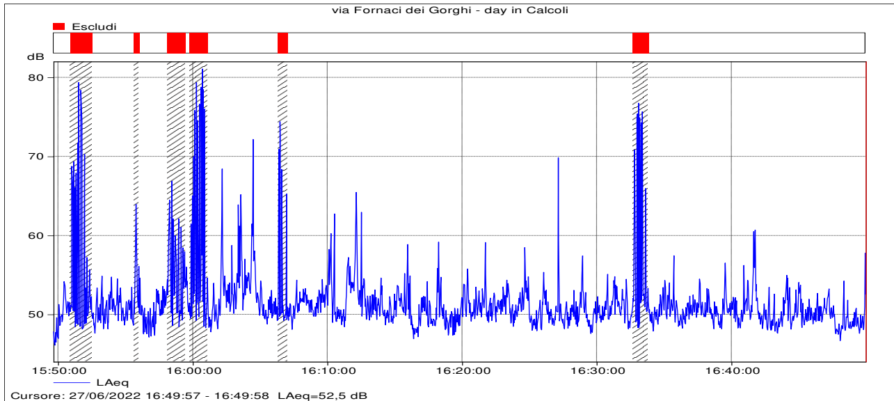
Fig.4.1.J- Centralina monitoraggio spot diurno – affaccio futura sottostazione – Time history livelli equivalenti (mascheramento: cani)
