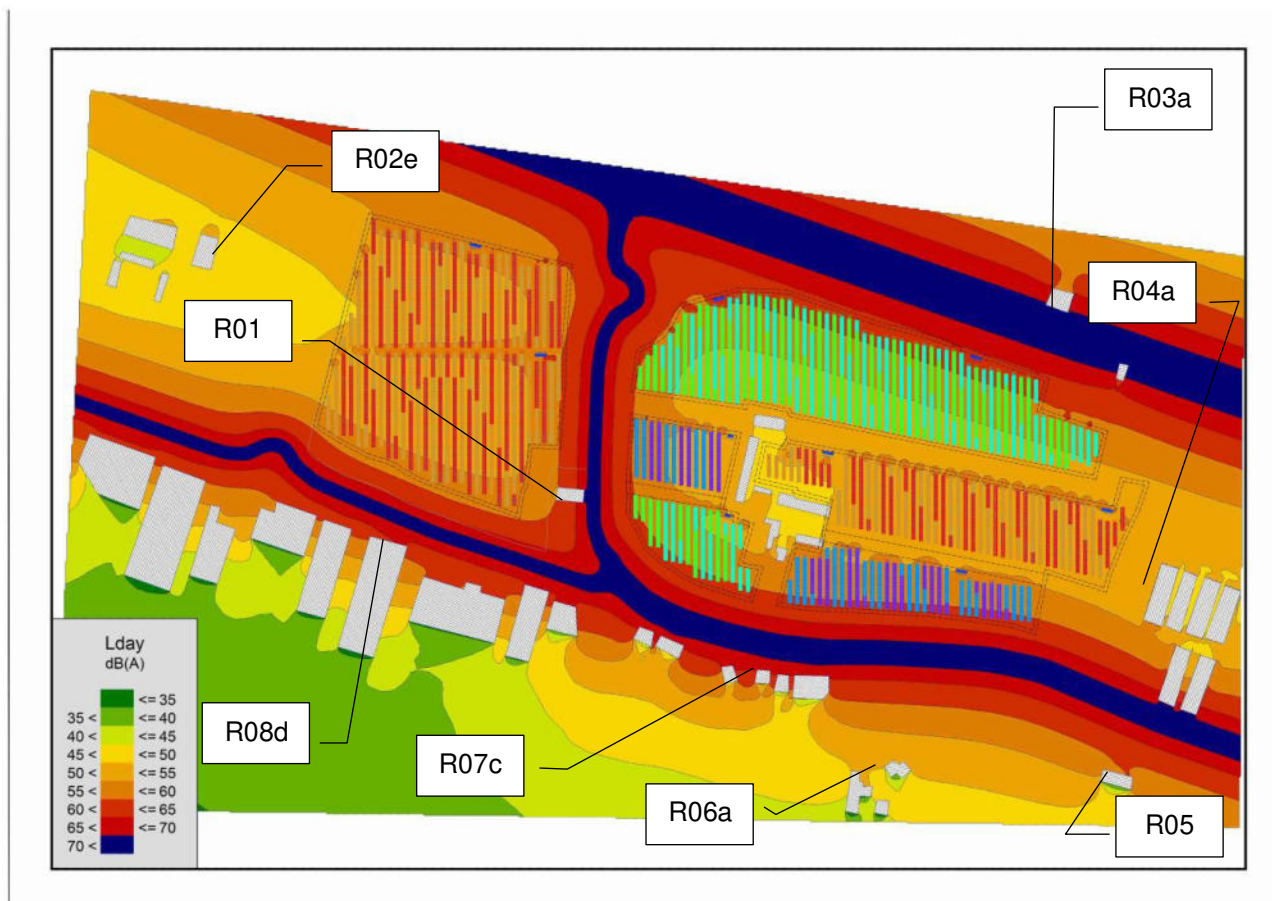
Fig.4.2.2.A – Modellazione scenario post operam - impianto agrivoltaico – restituzione livelli al continuo quota 4 m [dB(A)]
