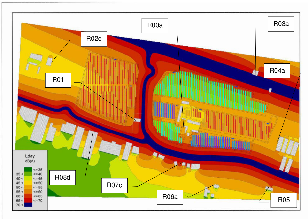
Fig.4.2.1.A – Modellazione scenario ante operam – impianto agrivoltaico – restituzione livelli al continuo quota 4 m [dB(A)]
