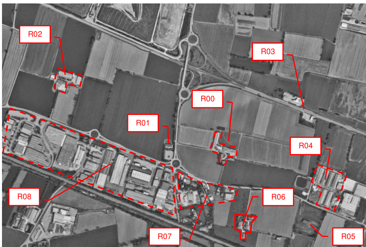
Fig.3.1.A – Localizzazione ricettori su foto aerea – impianto agrivoltaico
