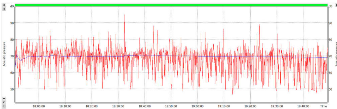
Fig.4.1.D – Centralina monitoraggio spot – affaccio SP 25 – Time history livelli equivalenti
