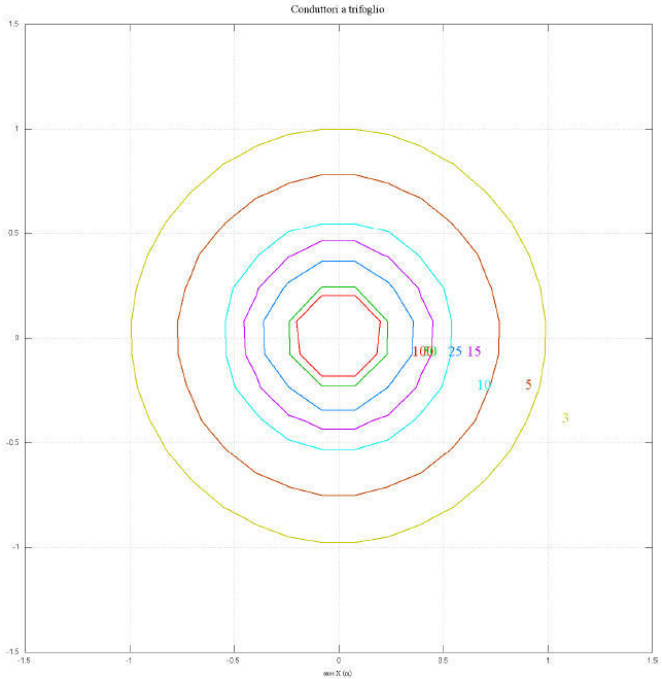
Figura 7.8: curve di equilivello per il campo magnetico linea MT in cavo elicordato interrata, calcolata con il software Magic prodotto da Be-Shielding s.r.l.
