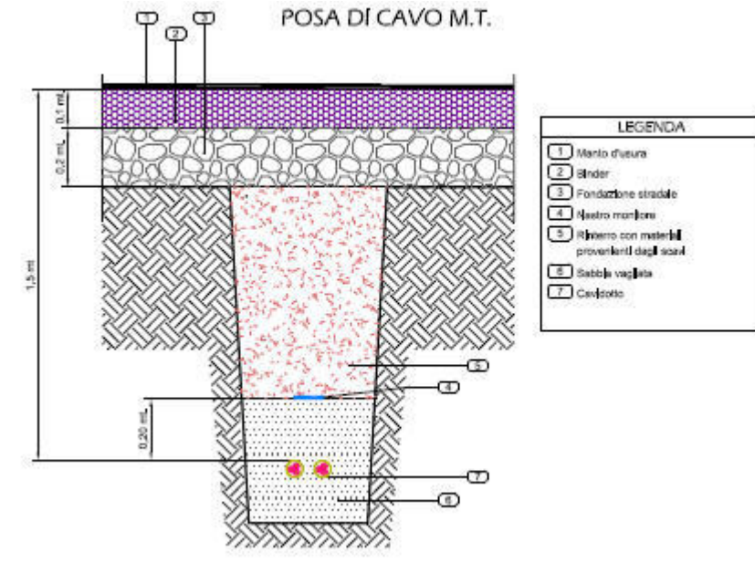
Figura 5.21: sezione tipo per l'interramento dei cavi MT.
