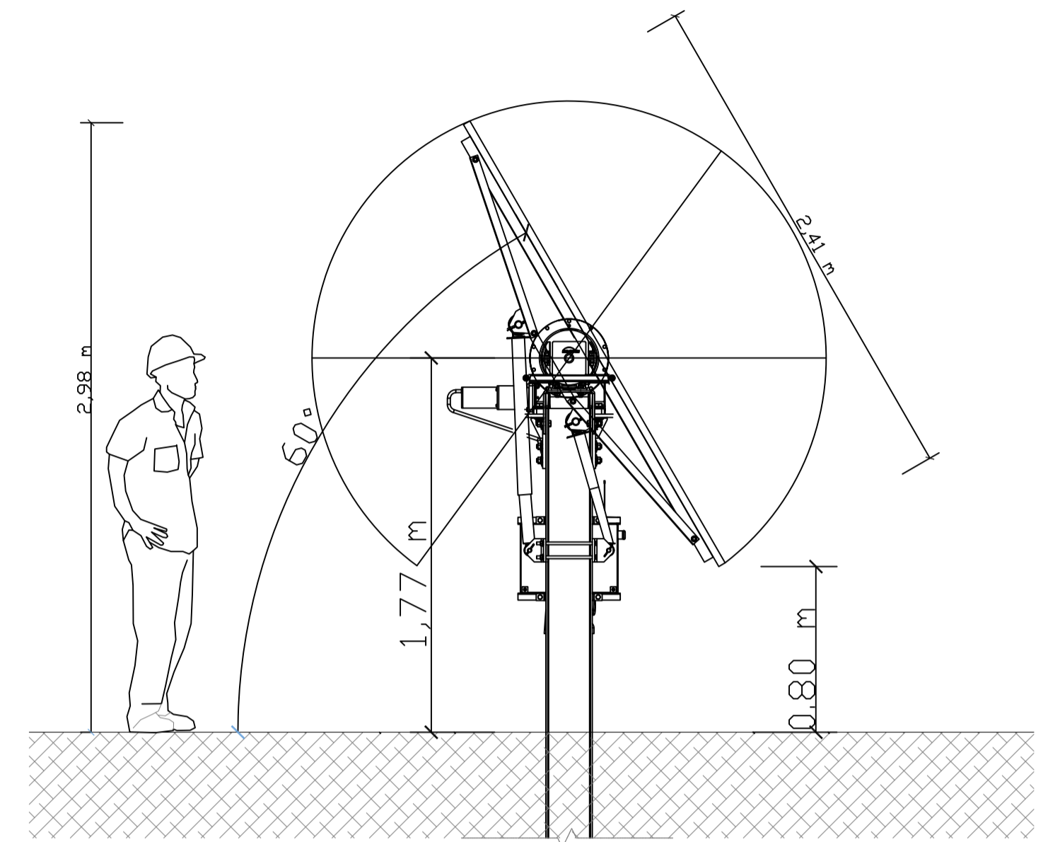
SISTEMA ROTAZIONE TRACKER +/-60°
