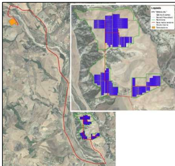
Figura 3: Layout di impianto (ortofoto)
