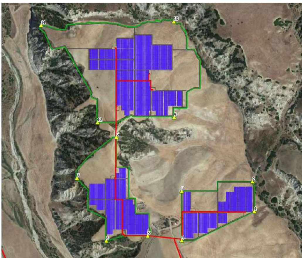
Figura n.4 - Coordinate dei vertici che racchiudono l'area dell'impianto fotovoltaico (ortofoto)
