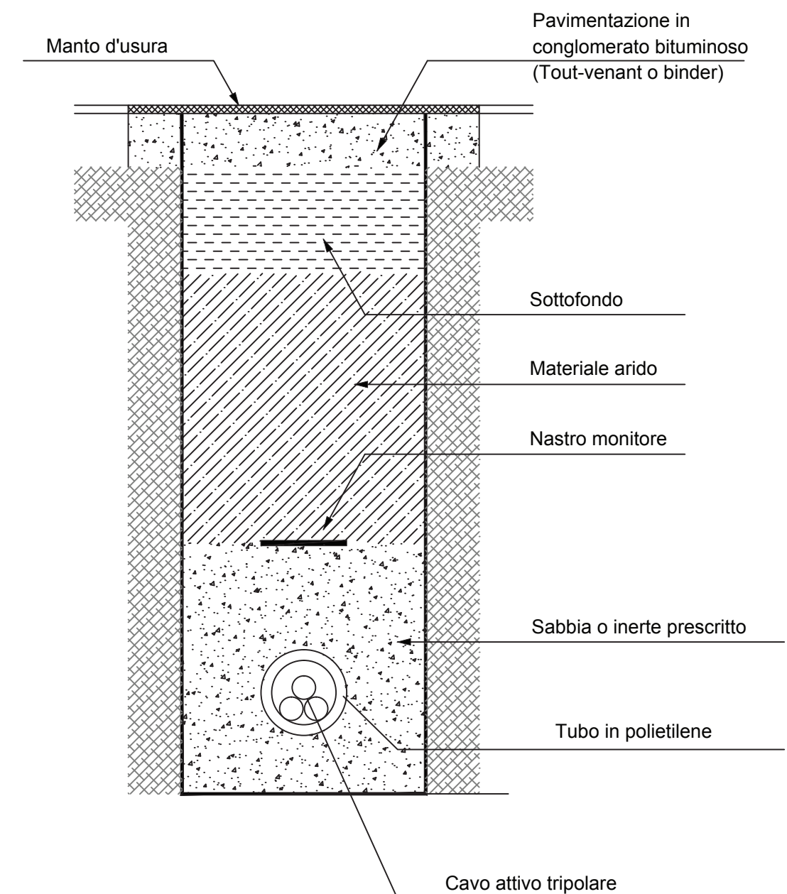
LINEA IN CAVO SOTTERRANEO IN TUBAZIONE POSA DI N.1 CAVI MT IN STRADA COMUNALE ASFALTATA
