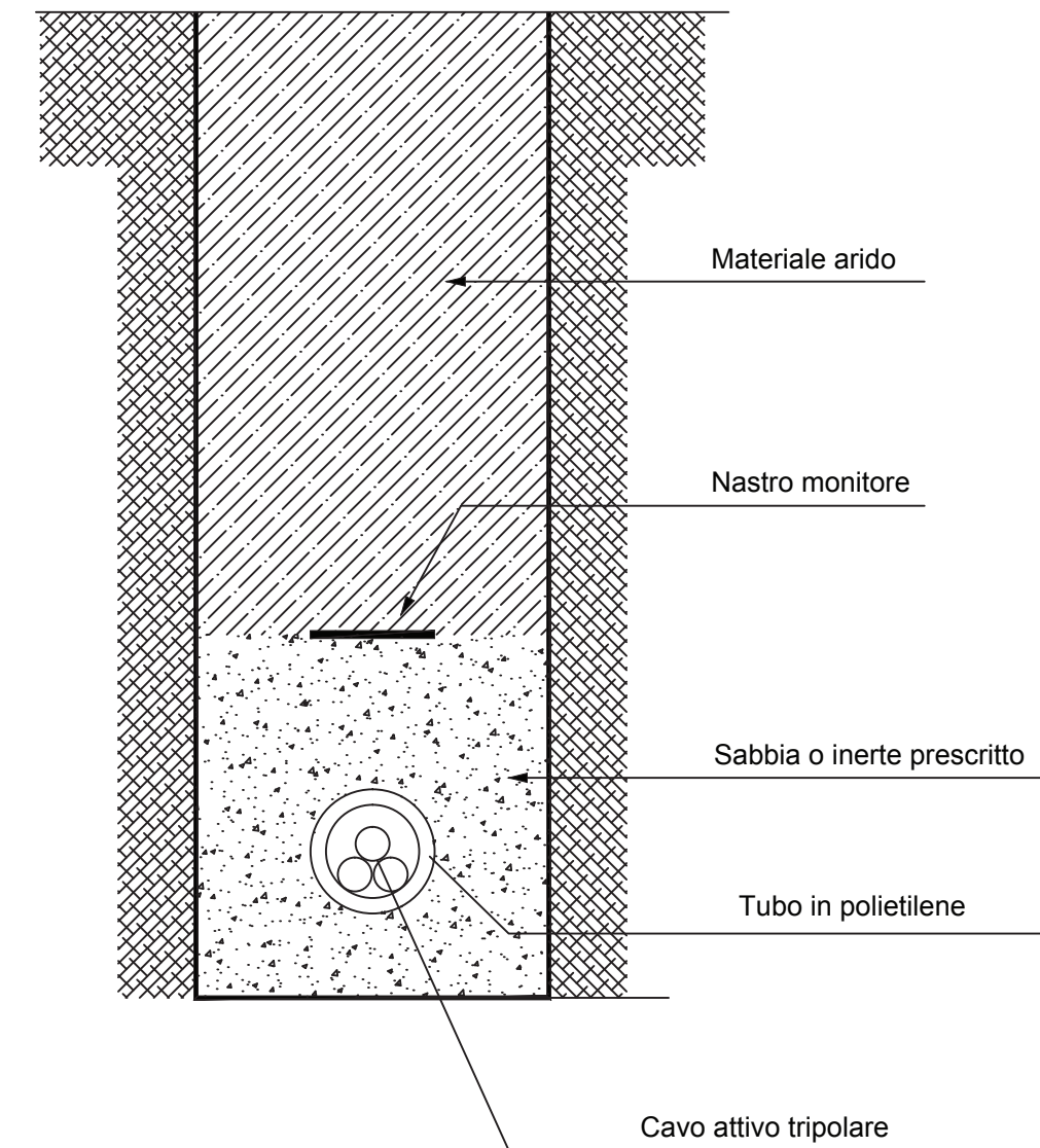
LINEA IN CAVO SOTTERRANEO IN TUBAZIONE POSA DI N.1 CAVI MT SU TERRENO NATURALE
