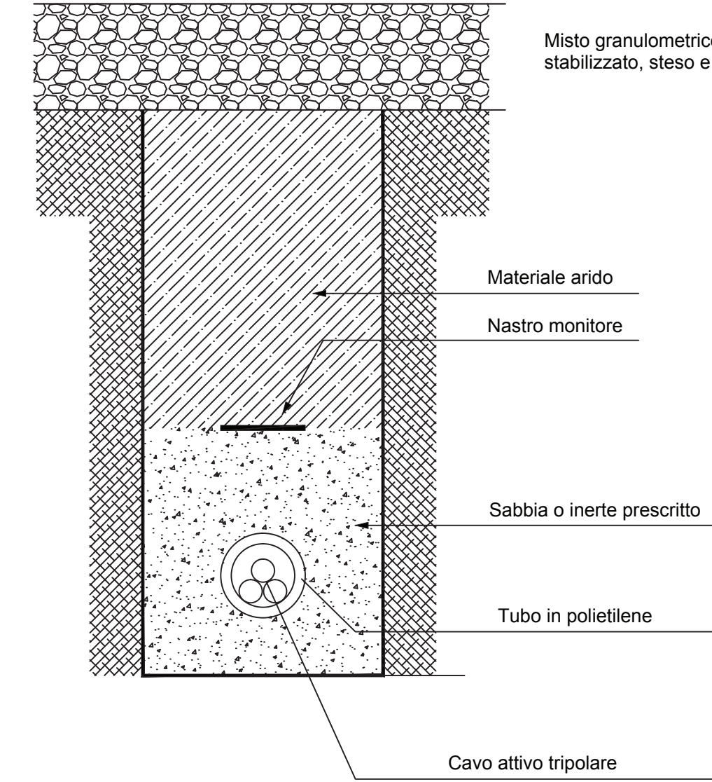
LINEA IN CAVO SOTTERRANEO IN TUBAZIONE POSA DI N.1 CAVI MT IN VIABILITÀ DI SERVIZIO SU MISTO STABILIZZATO
