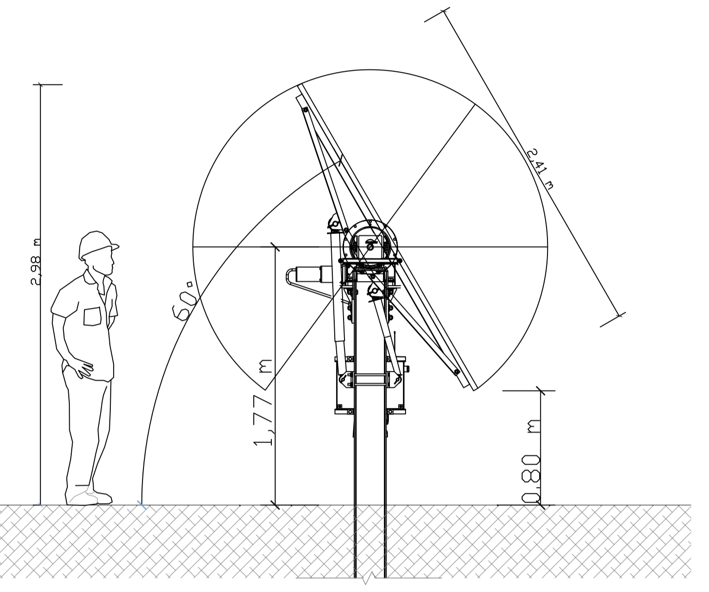
SISTEMA ROTAZIONE TRACKER +/-60°
