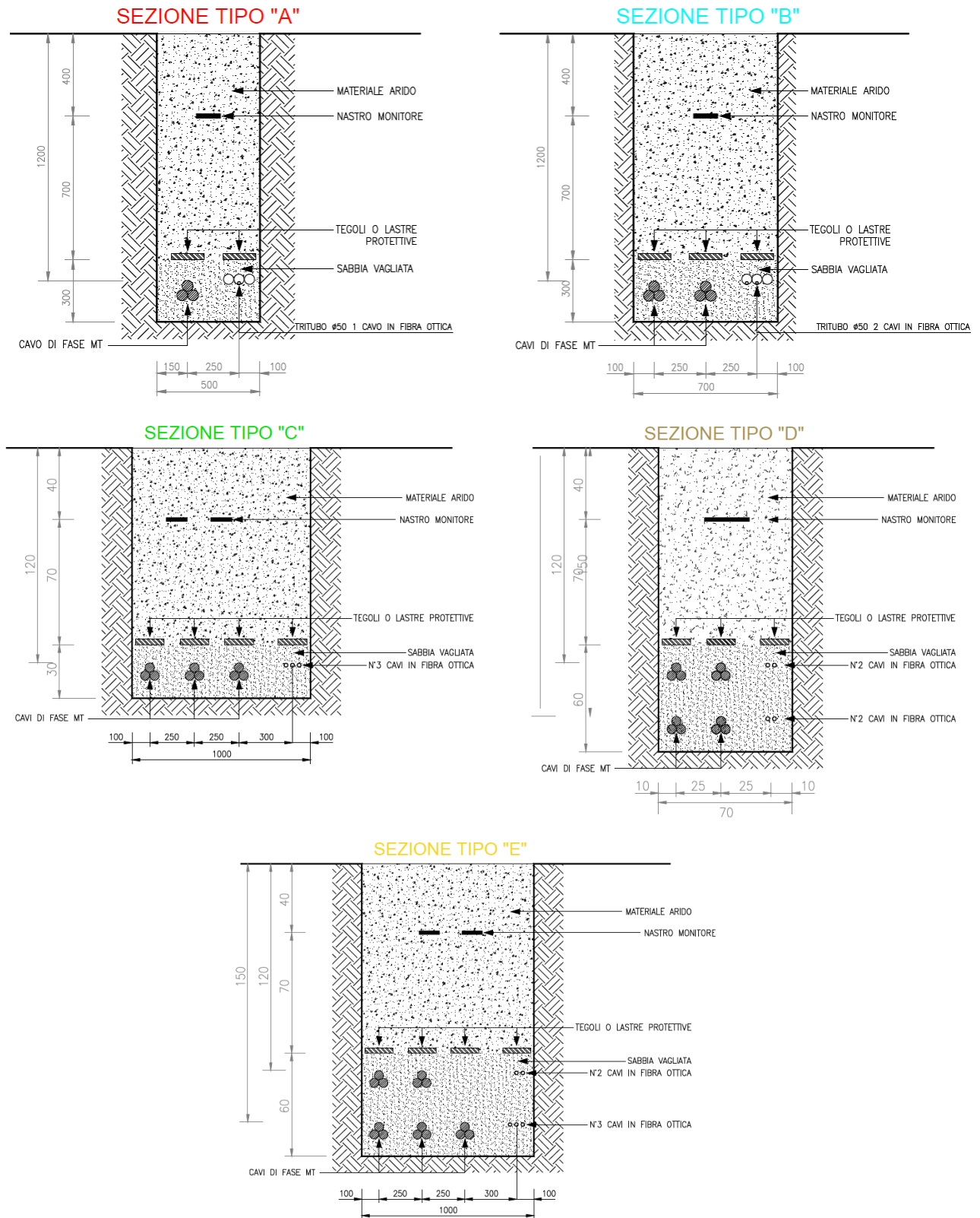
Figura 1: Sezione tipica di posa della linea in cavo su strade sterrate
