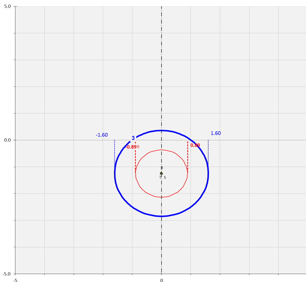
Figura 9: Curve di equilivello per il campo di induzione magnetica generato dalla linea MT (Sezione 1 – una terna MT)
