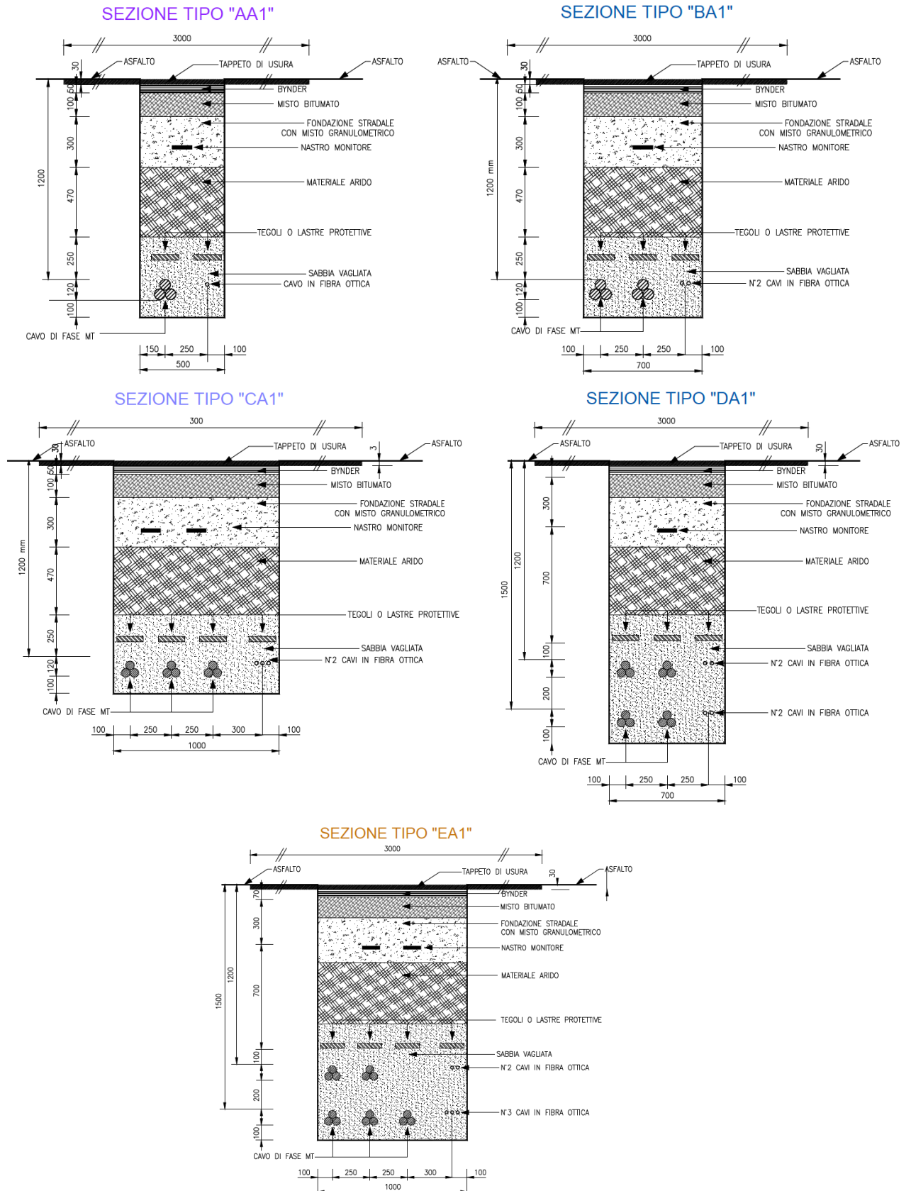
Figura 3: Sezione tipica di posa della linea in cavo su sede stradale
