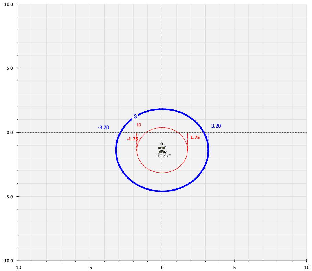
Figura 12: Curve di equilivello per il campo di induzione magnetica generato dalla linea MT (Sezione 4 – quattro terne MT)
