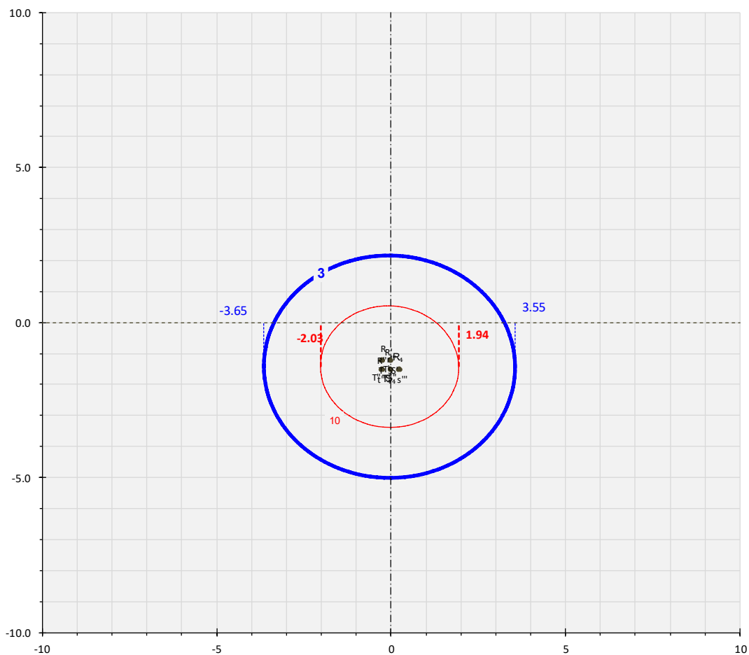
Figura 13: Curve di equilivello per il campo di induzione magnetica generato dalla linea MT (Sezione 5 – cinque terne MT)
