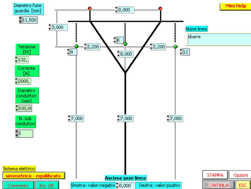
Figura 15: Linea AT con disposizione conduttori in piano assimilabile ad un sistema semplice sbarra a 132/150 kV
