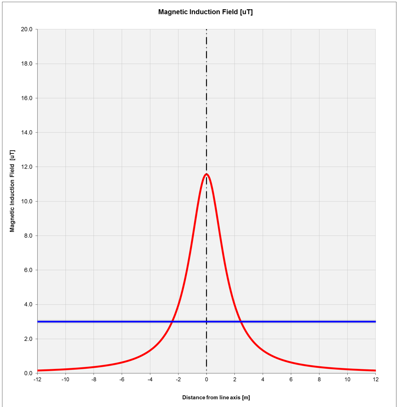
Figura 17: Andamento dell'induzione magnetica prodotta dalla linea in cavo AT
