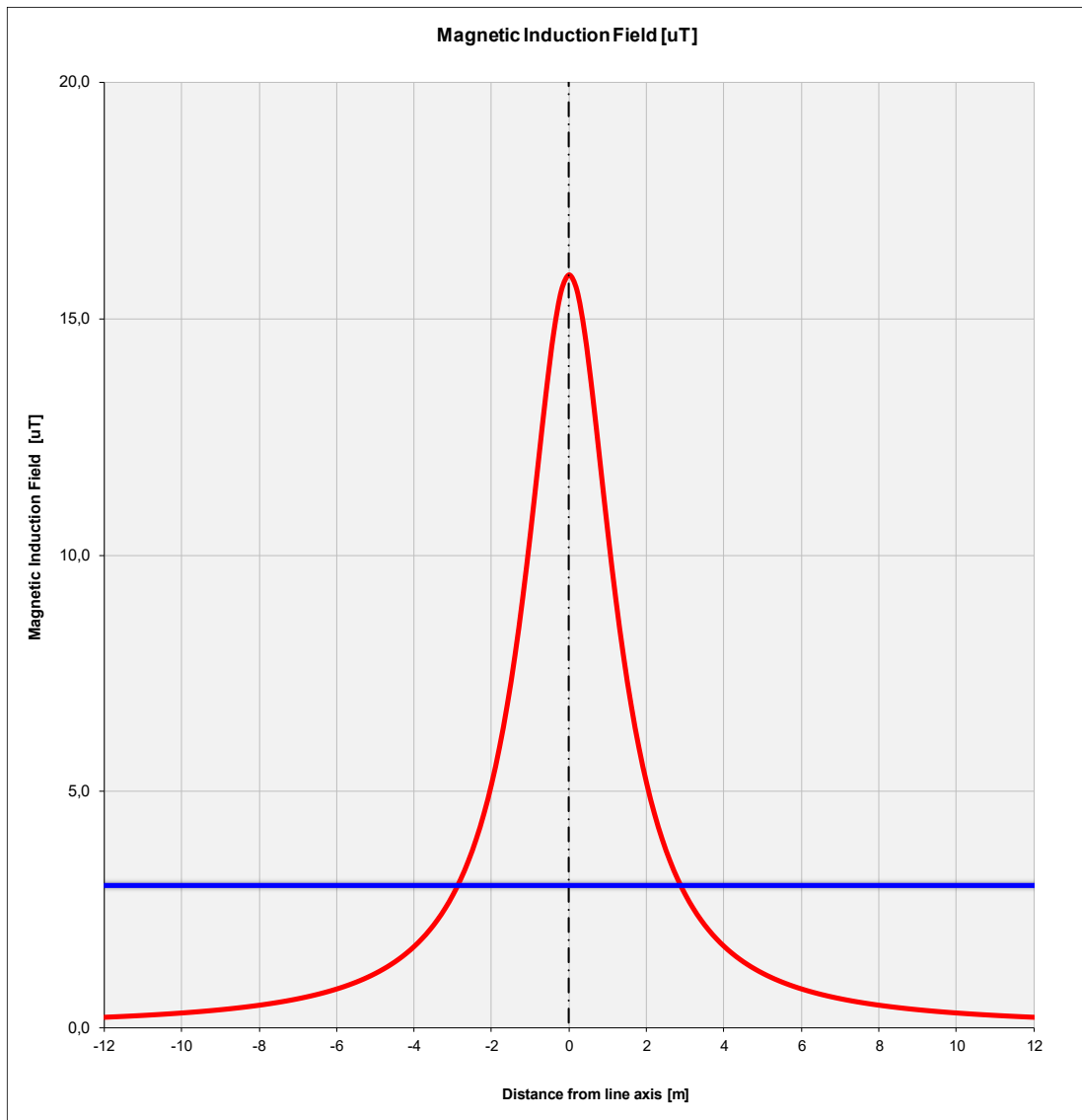
Figura 7: Andamento dell'induzione magnetica prodotta dalla linea in cavo per la sezione 4 (quattro terne MT)
