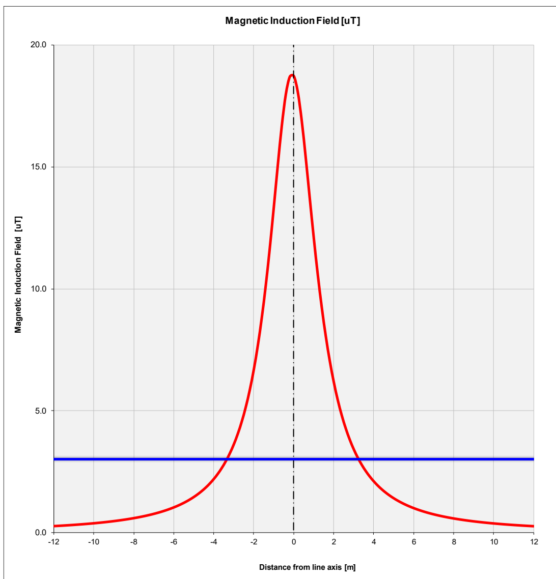
Figura 8: Andamento dell'induzione magnetica prodotta dalla linea in cavo per la sezione 5 (cinque terne MT)
