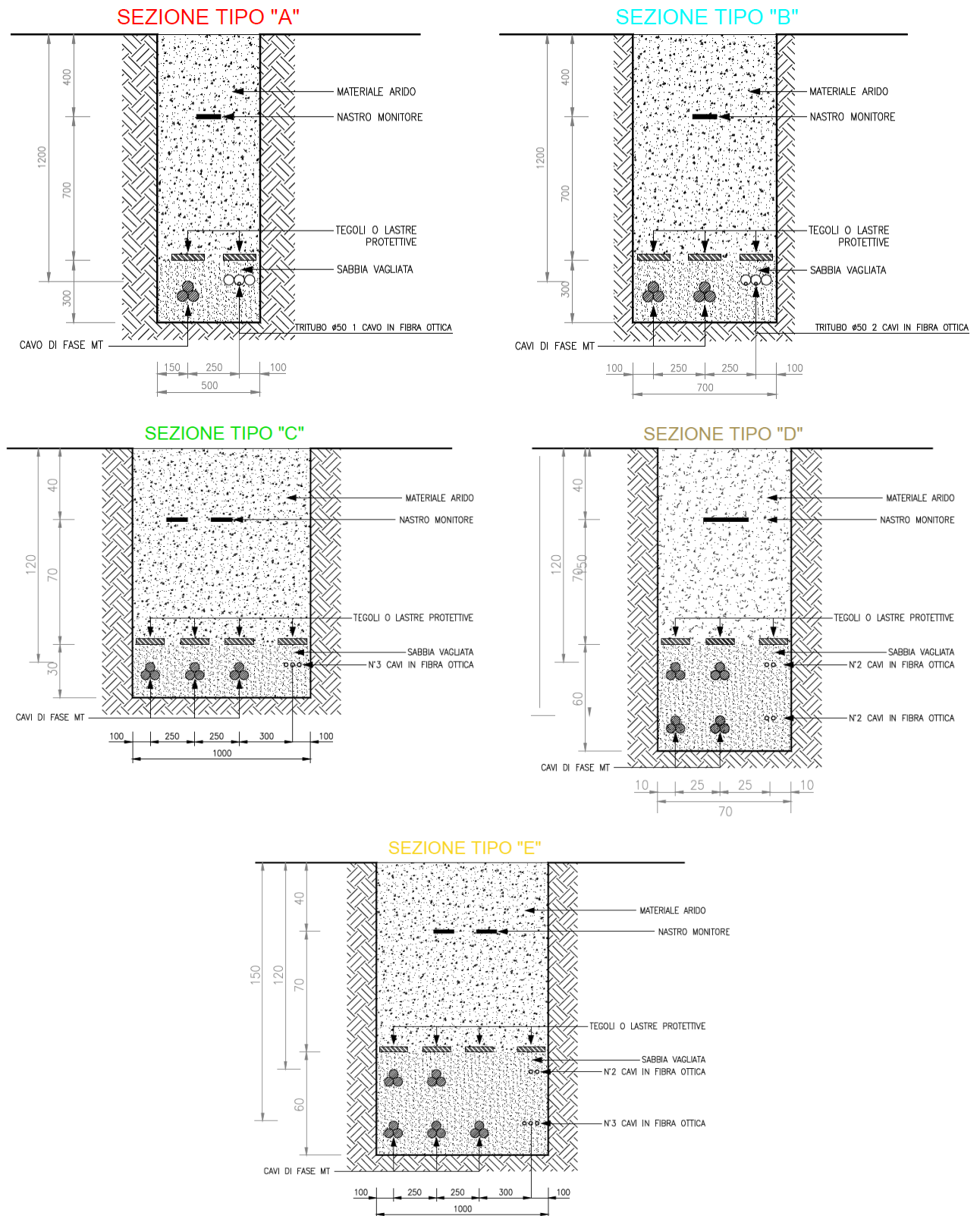
Figura 2: Sezione tipica di posa della linea in cavo su strade sterrate
