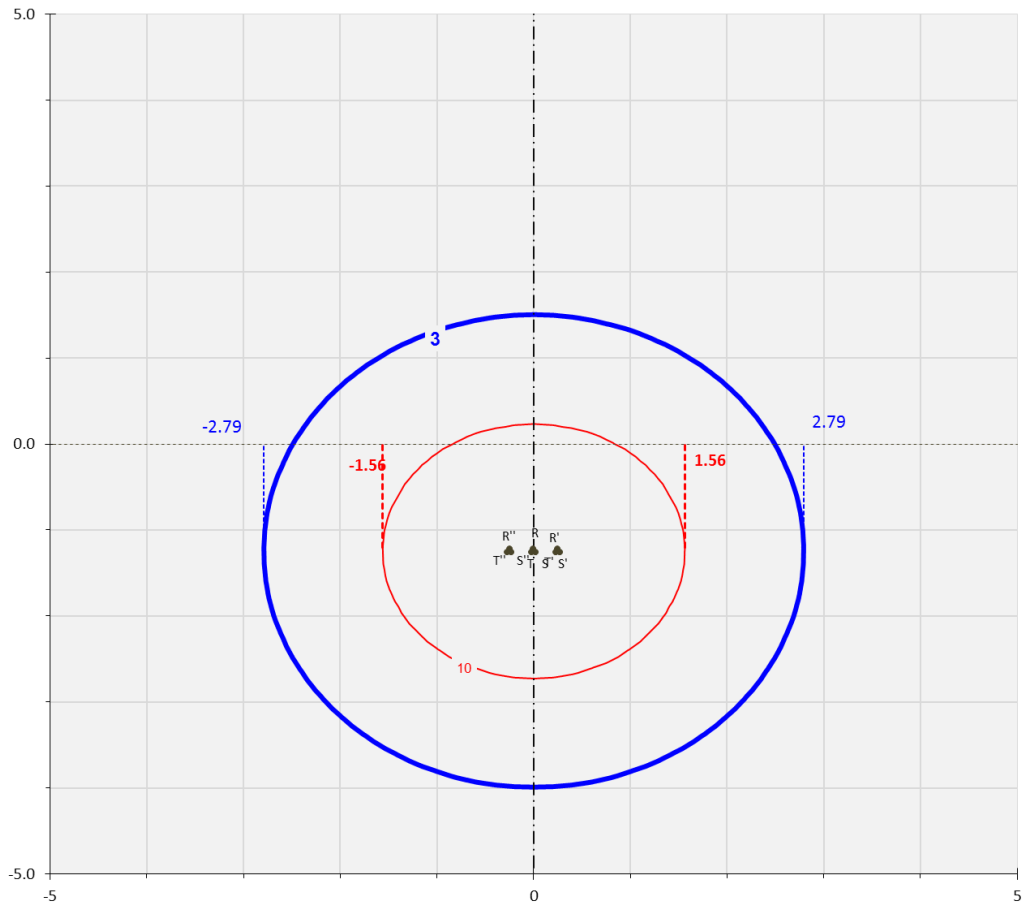
Figura 11: Curve di equilivello per il campo di induzione magnetica generato dalla linea MT (Sezione 3 – tre terne MT)
