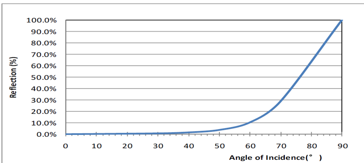
Figura 3 - Rapporto tra percentuale di riflessione e angolo di incidenza, della luce solare
