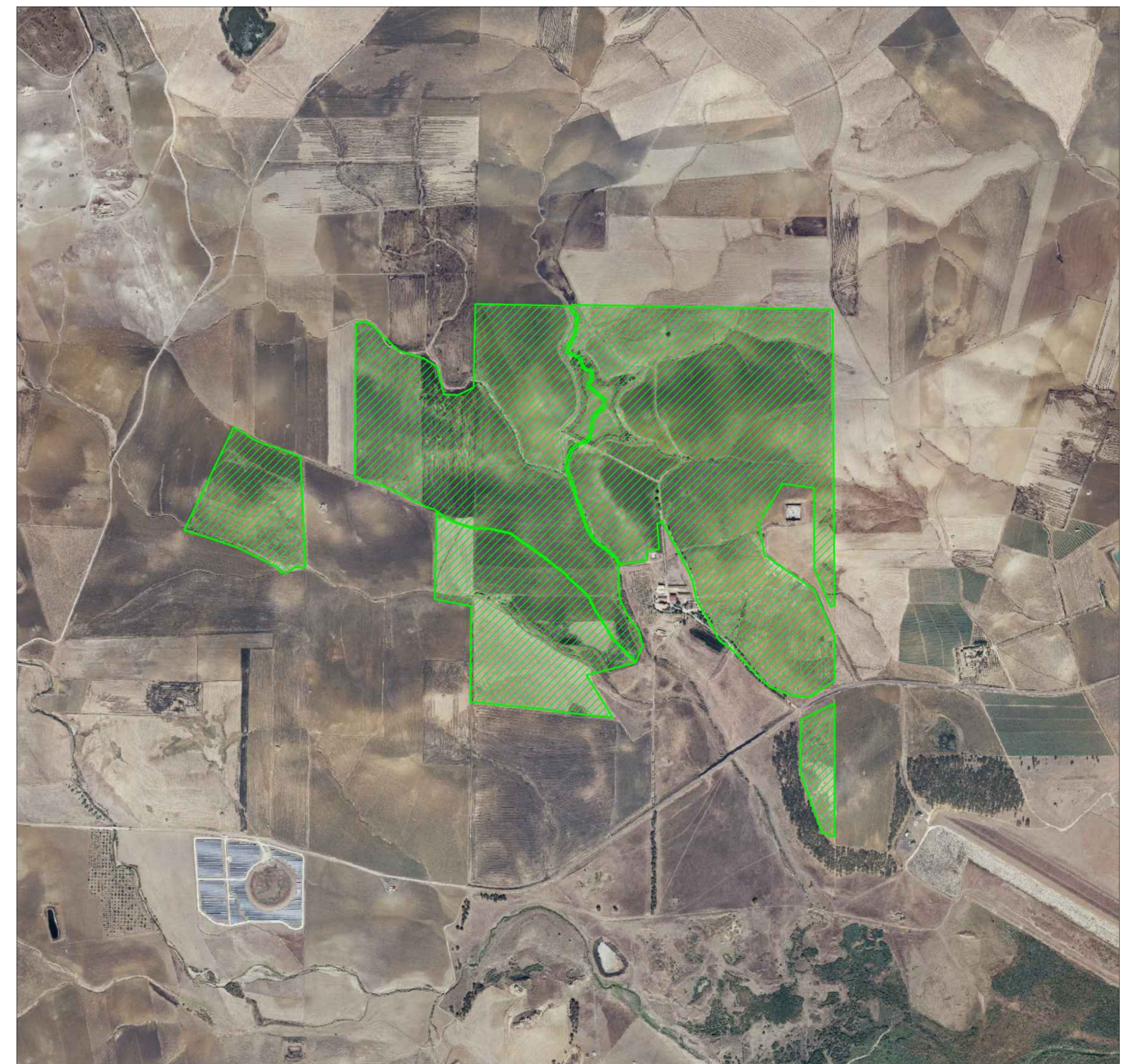
Area Impianto FV in progetto
