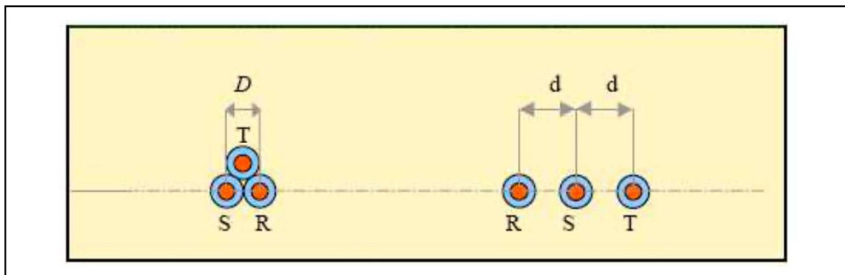
Figura 4-4 Modalità di posa cavo AT
