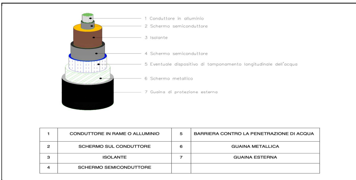
Figura 4-3 caratteristiche tecniche Cavo AT per trasporto energia
