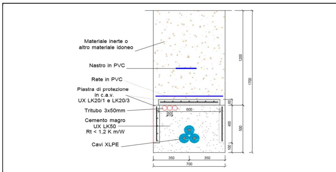
Figura 4-5 Particolare di Posa Cavidotto AT
