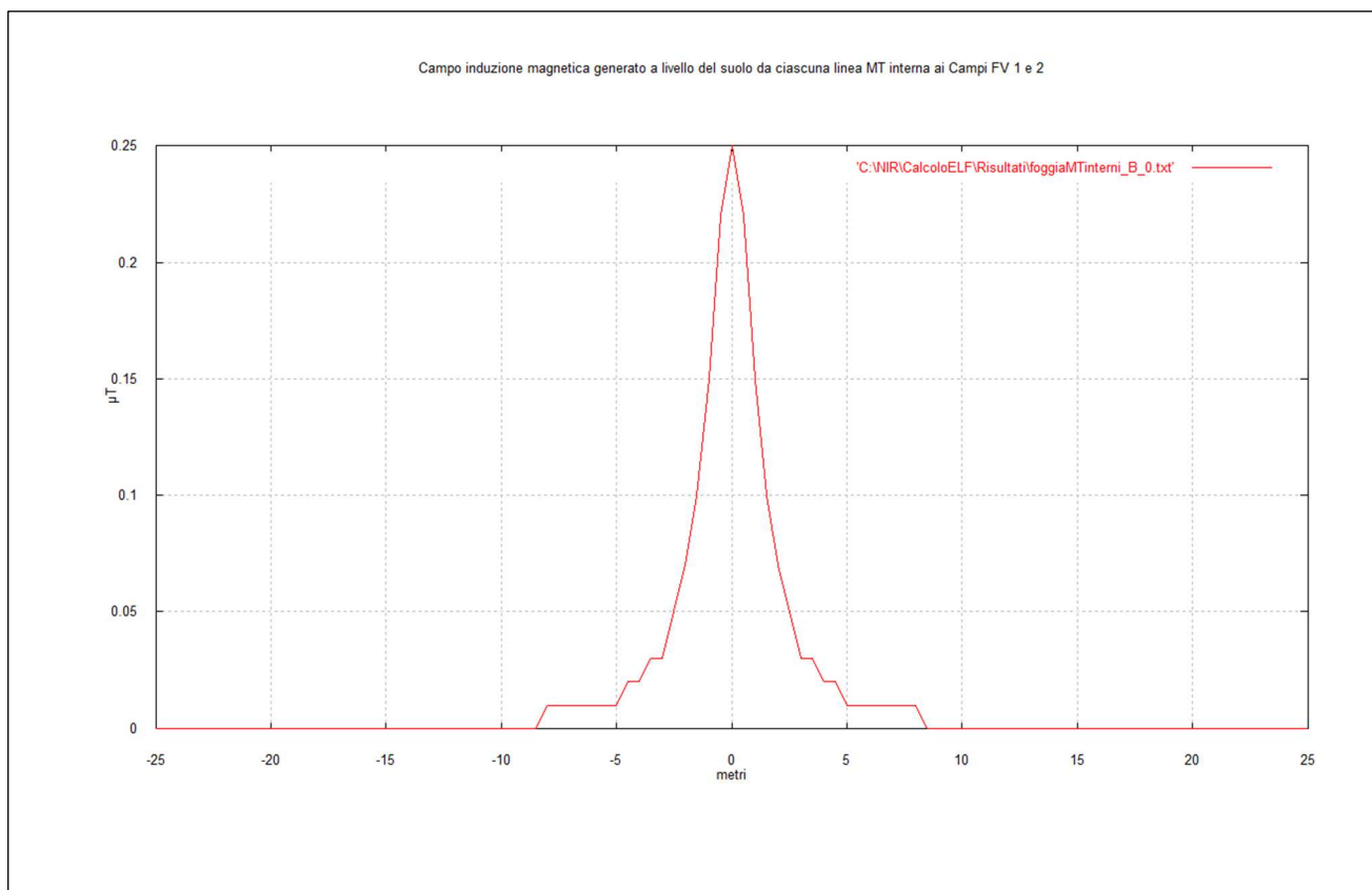
Grafico rappresentativo campo di induzione magnetica generati dai cavidotti MT a 30KV interni ai campi Fotovoltaici.
