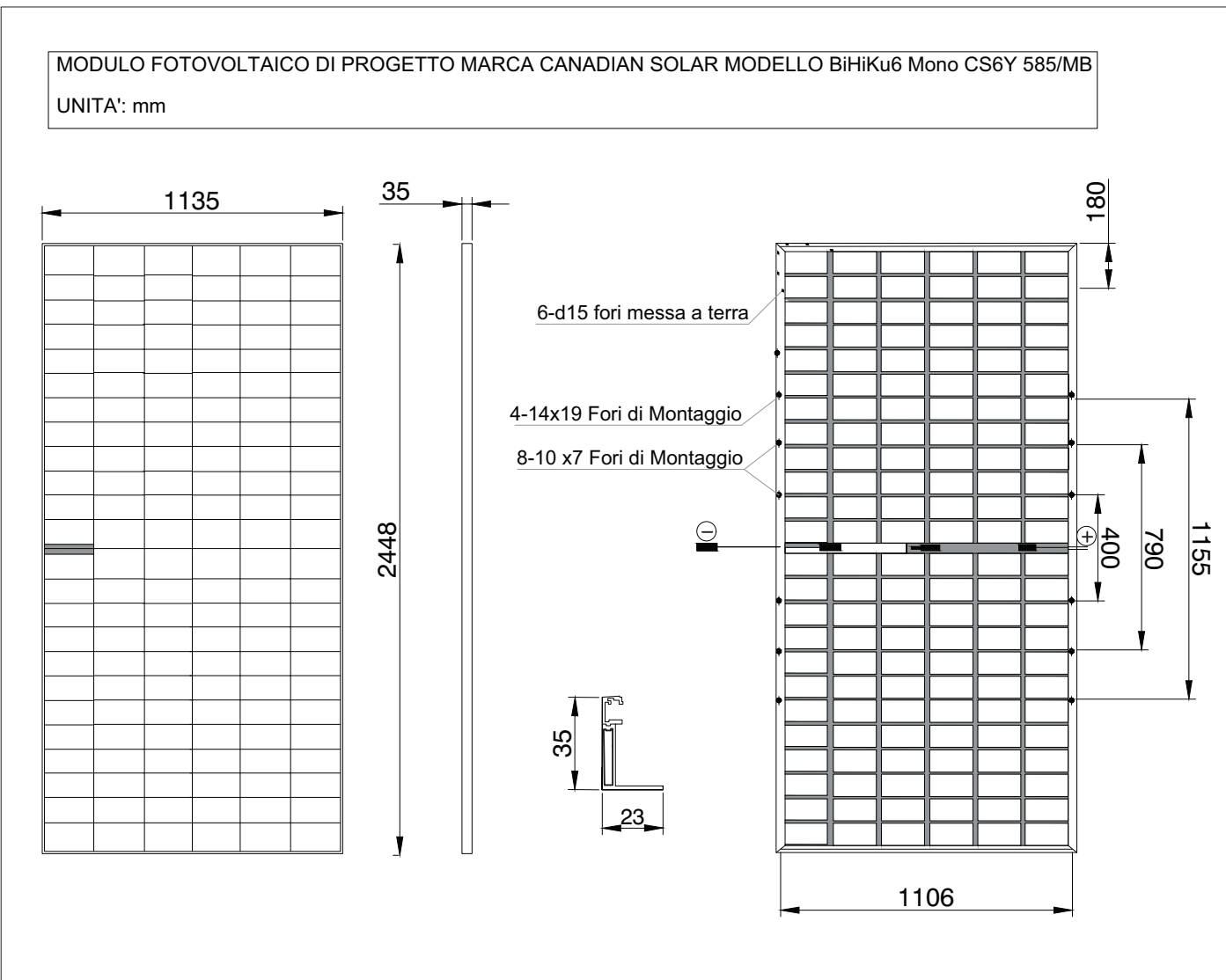
Particolare Modulo Utilizzato - Scala 1: 25
