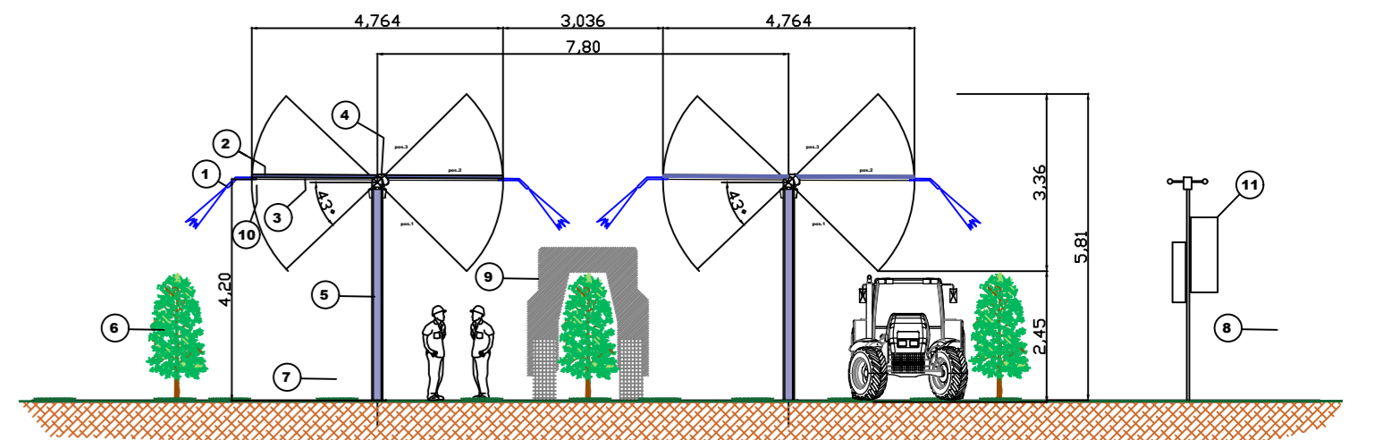
Schema TRAKER Tipologia impianto AFV
