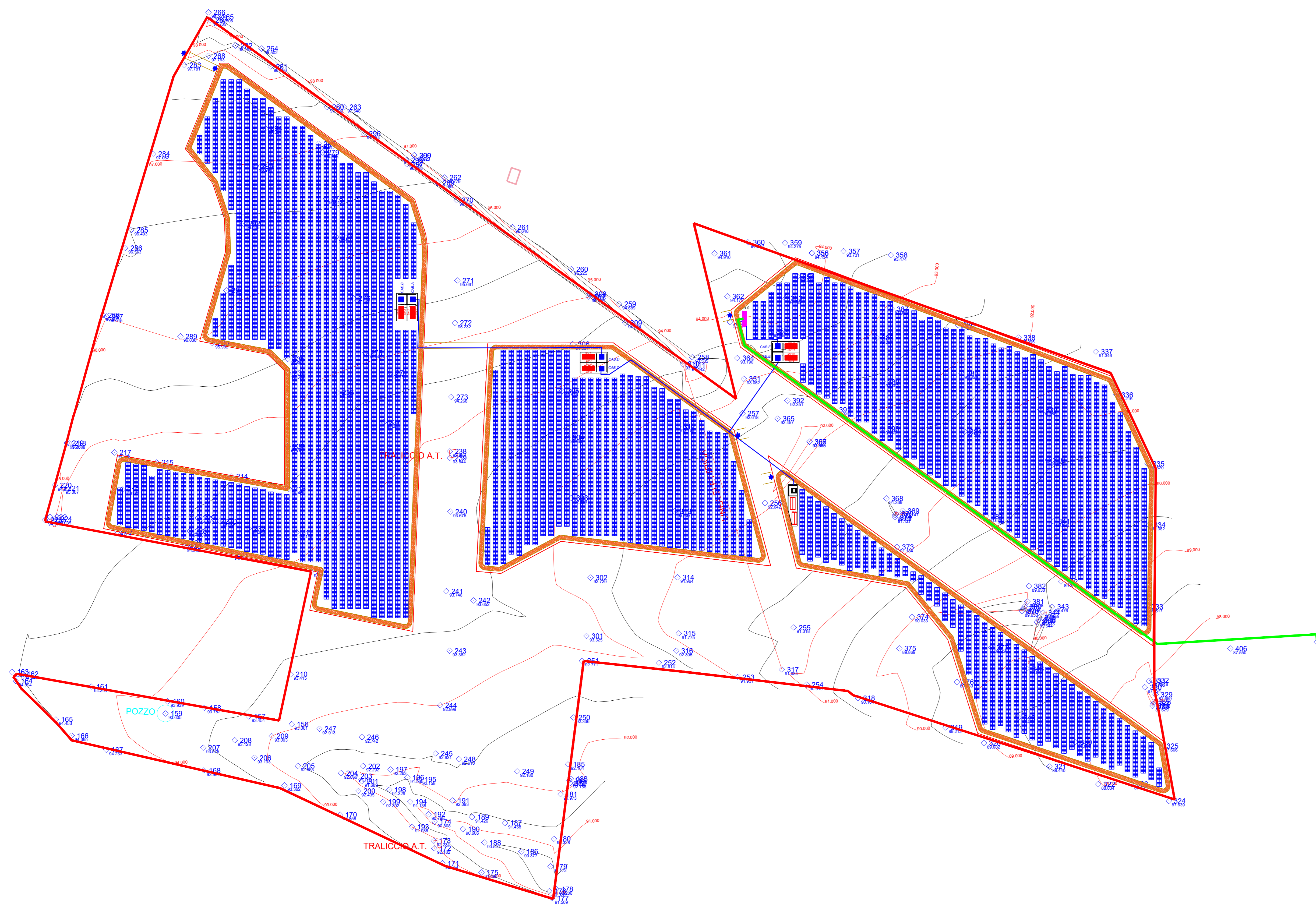
AREA CABINA Scala 1:2000
