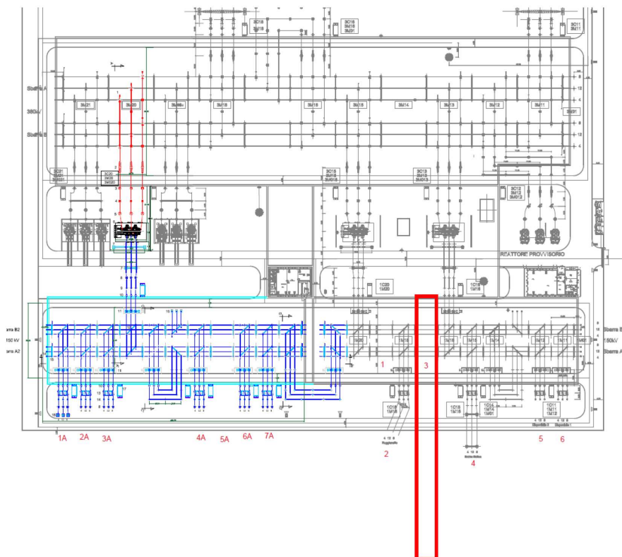
Stazione TERNA ERCHIE - Stallo in 150 kV
