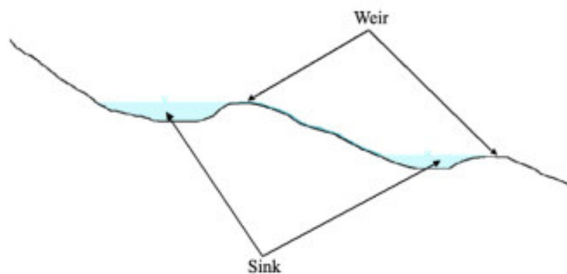
Fig. 3.3 – Profilo schematico di un bacino con serbatoi multipli e deflusso che si attiva per stramazzo rispetto ad una soglia morfologica (figura estratta da: RATIONALE FOR FLOOD PREDICTION IN KARST ENDORHEIC AREAS (2014) – V. Iacobellis, A. Castorani, A. R. Di Santo, A. Gioia. Journal of Arid Environments XXX (2014) 1-11.
