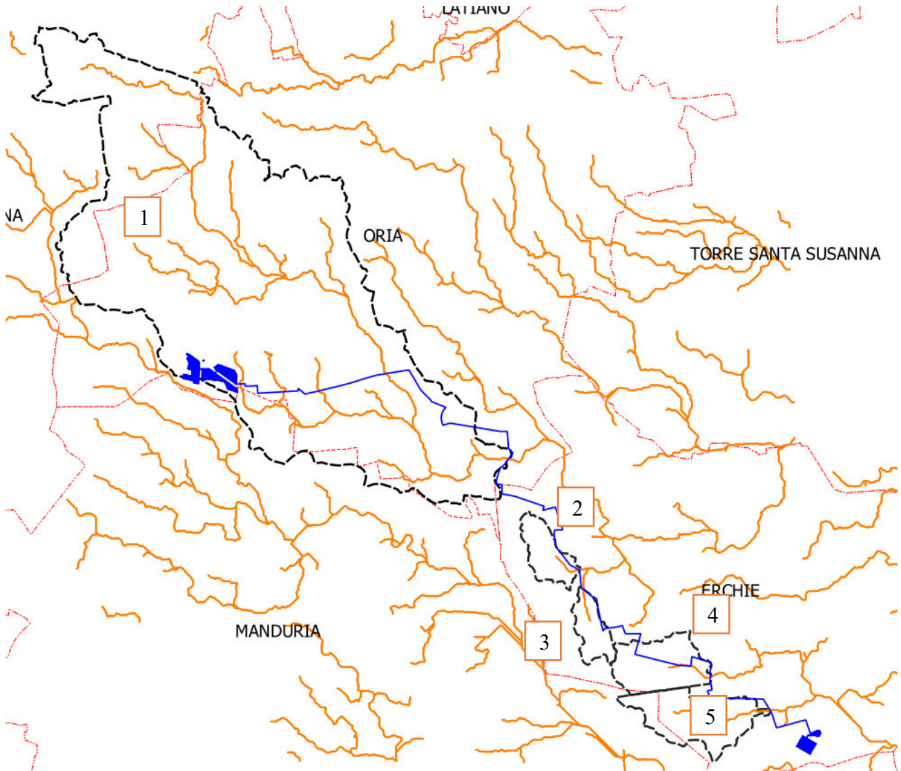
Fig. 4.1 - Interferenze con la rete idrografica e perimetrazione dei bacini di progetto
