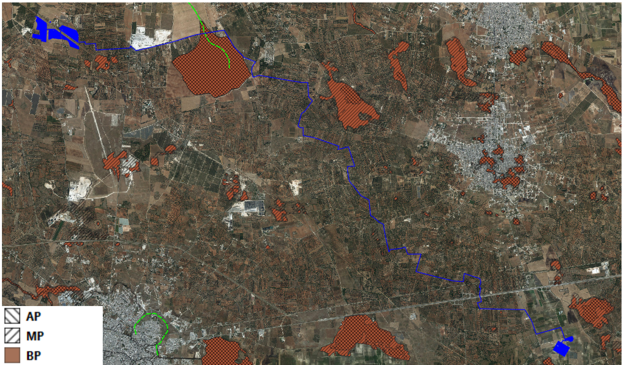
Fig. 4.2 – Interferenze tra gli interventi di progetto e le aree a pericolosità idraulica e la rete idrografica (estratta dalla Carta idrogeomorfologica)
