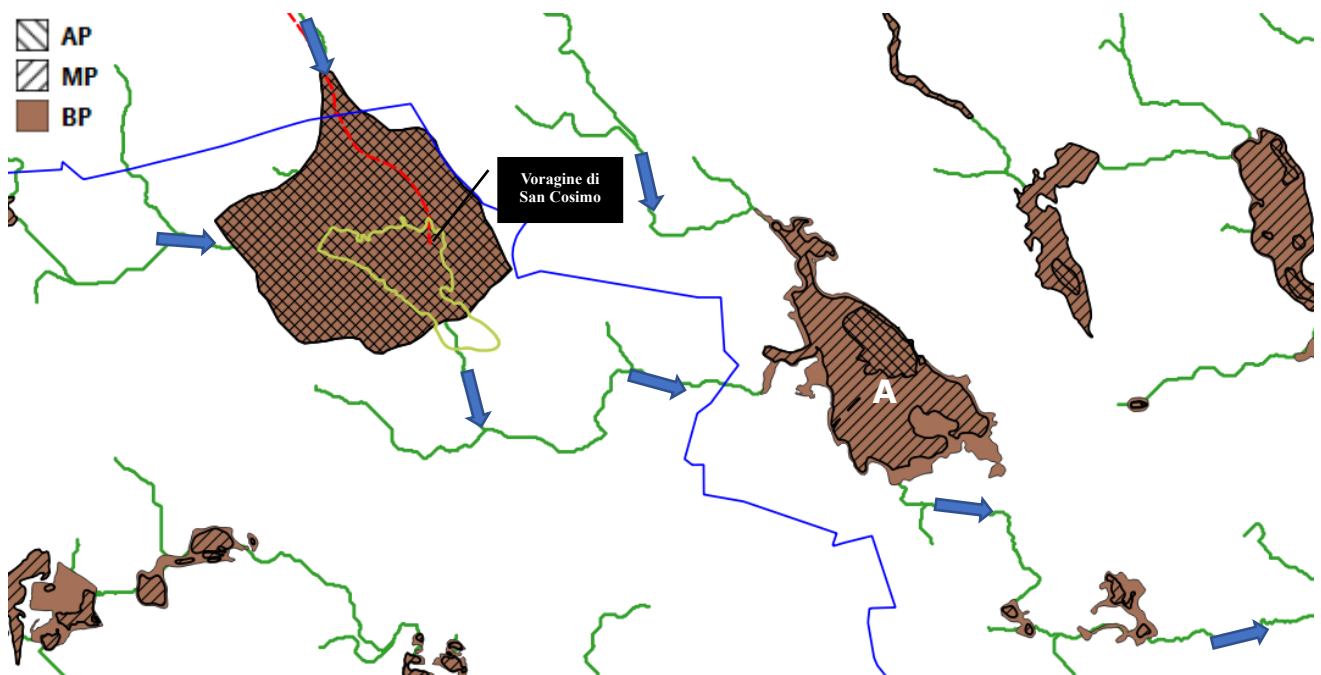
Fig. 4.3 – Schema idrografico relativo alla parte di valle del bacino 1; in blu è riportato il tracciato del cavidotto, in verde la rete idrografica estratta dal DTM Puglia (le frecce celesti indicano il verso di deflusso), in rosso la rete idrografica riportata sulla Carta idrogeomorfologica. Il perimetro della conca alluvionale che contiene la Voragine di San Cosimo e indicato in giallo
