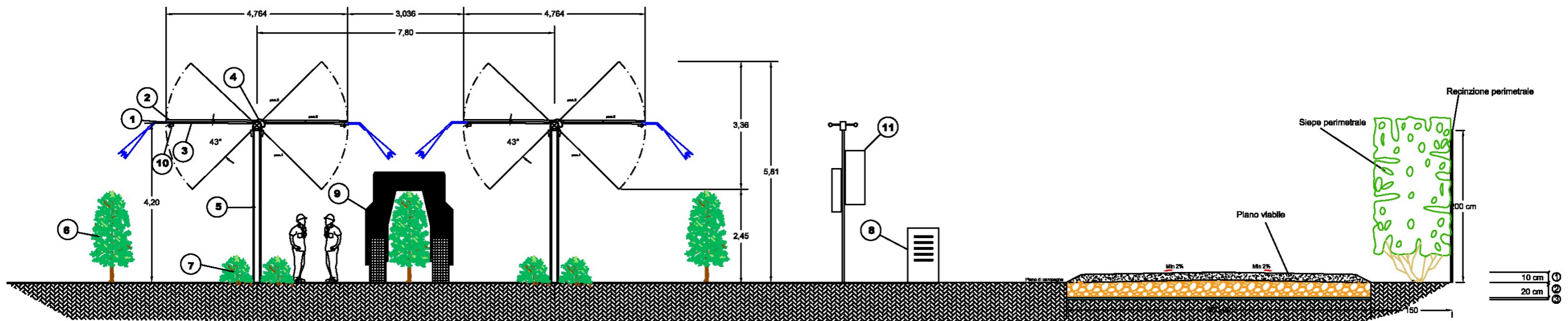
Schema TRAKER Tipologia impianto AFV
