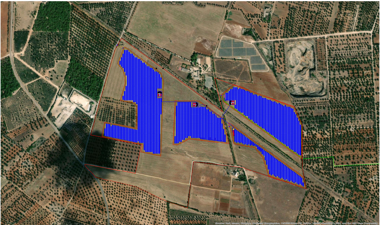
Impianto AFV con coltivazione agronomica
