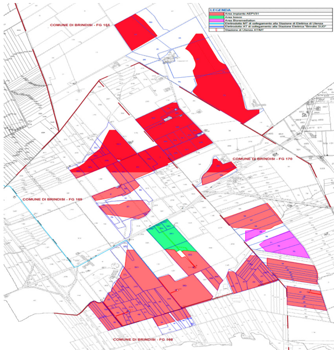
Tavola n. 1: Impianto suddiviso in campi e sottocampi fotovoltaici.
