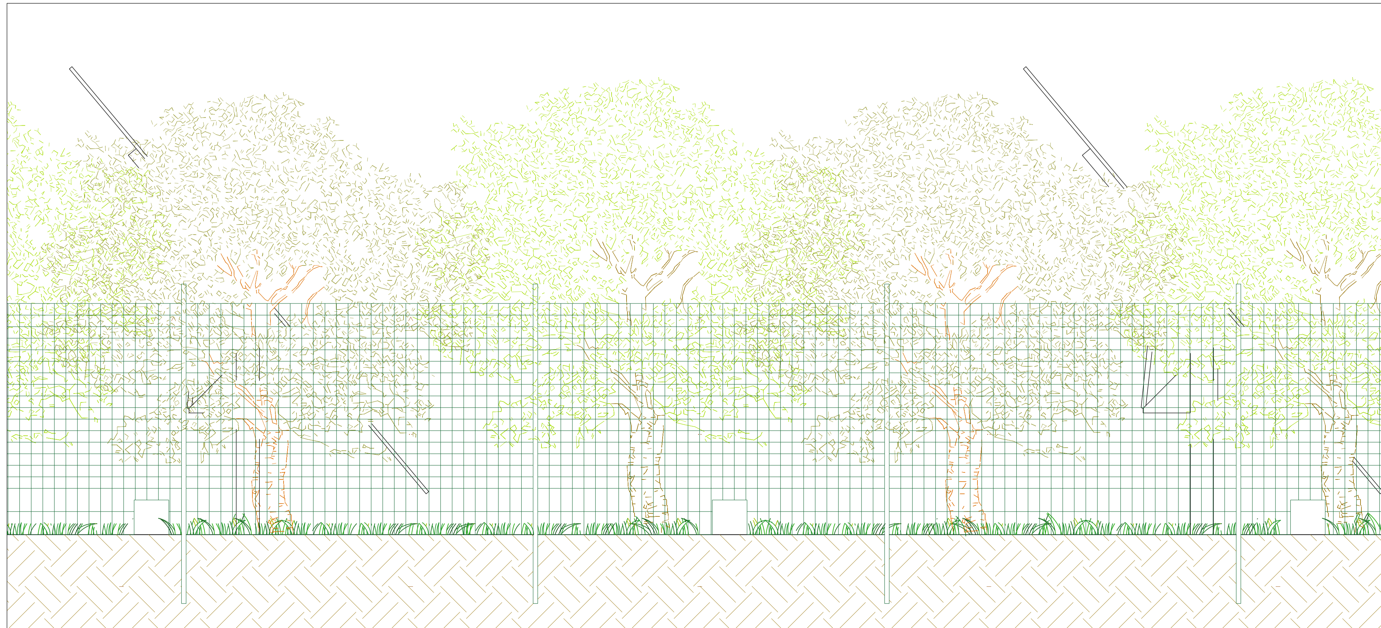
PARTICOLARE COSTRUTTIVO RECINZIONE PERIMETRALE - scala 1:20
