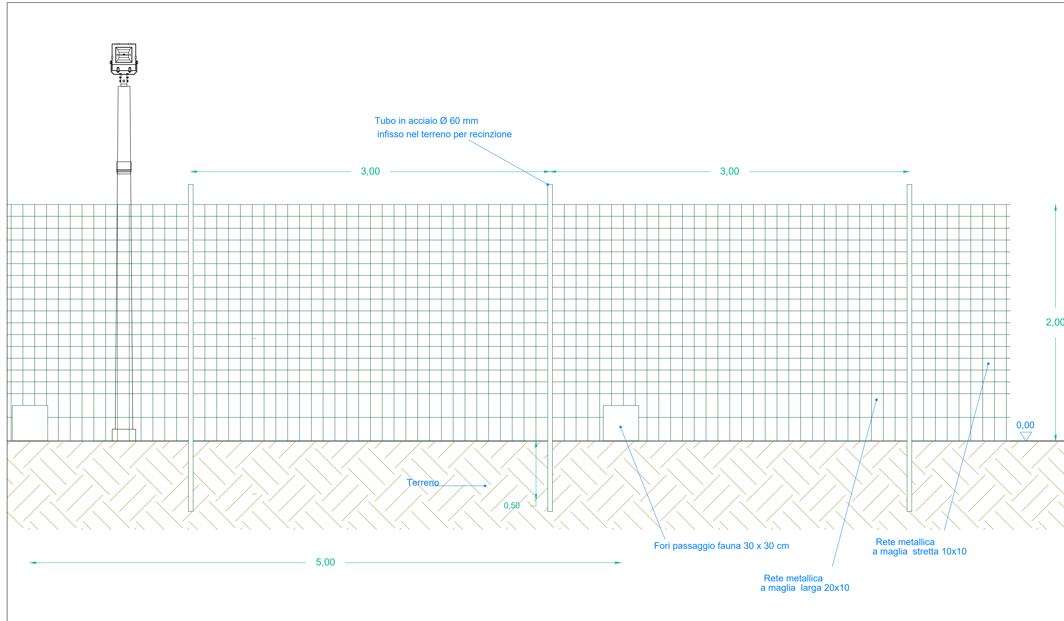
PARTICOLARE COSTRUTTIVO RECINZIONE PERIMETRALE - scala 1:20
