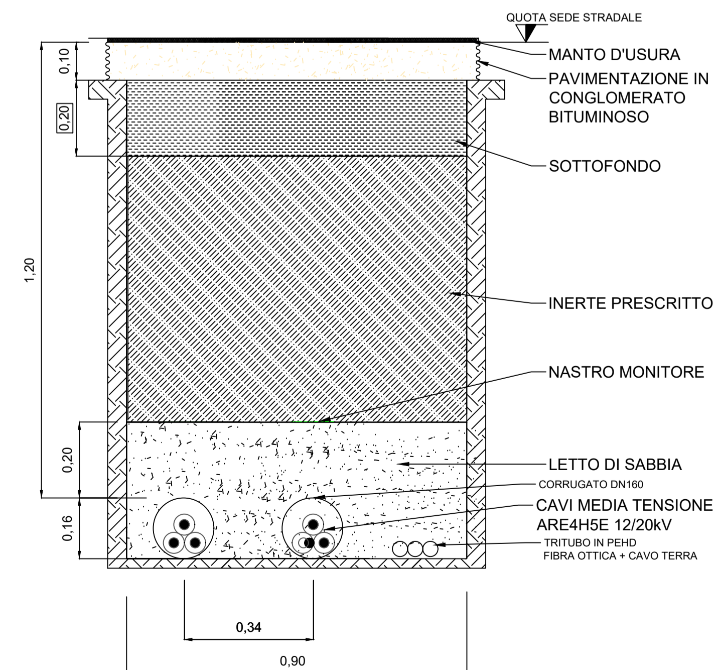
CAVIDOTTO TIPO MT DI CONNESSIONE IN STRADA SCALA 1:10
