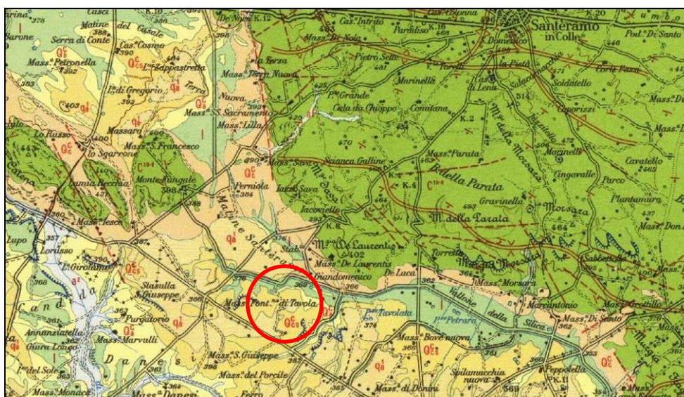
Carta Geologica d'Italia (Stralcio F° 189 Altamura)
