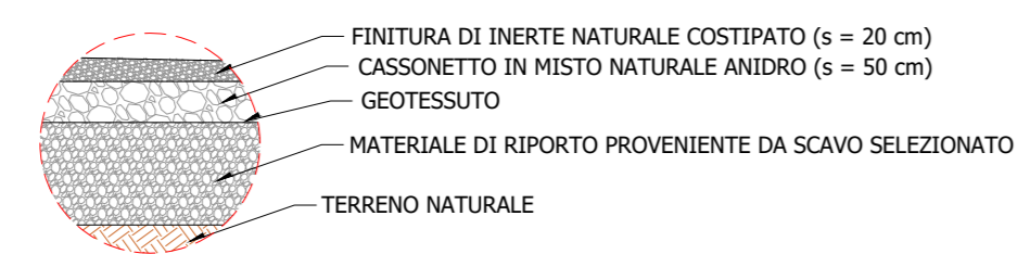
Particolare 1 - Struttura stradale scala 1:50
