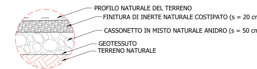
Particolare 2 - Struttura stradale scala 1:50
