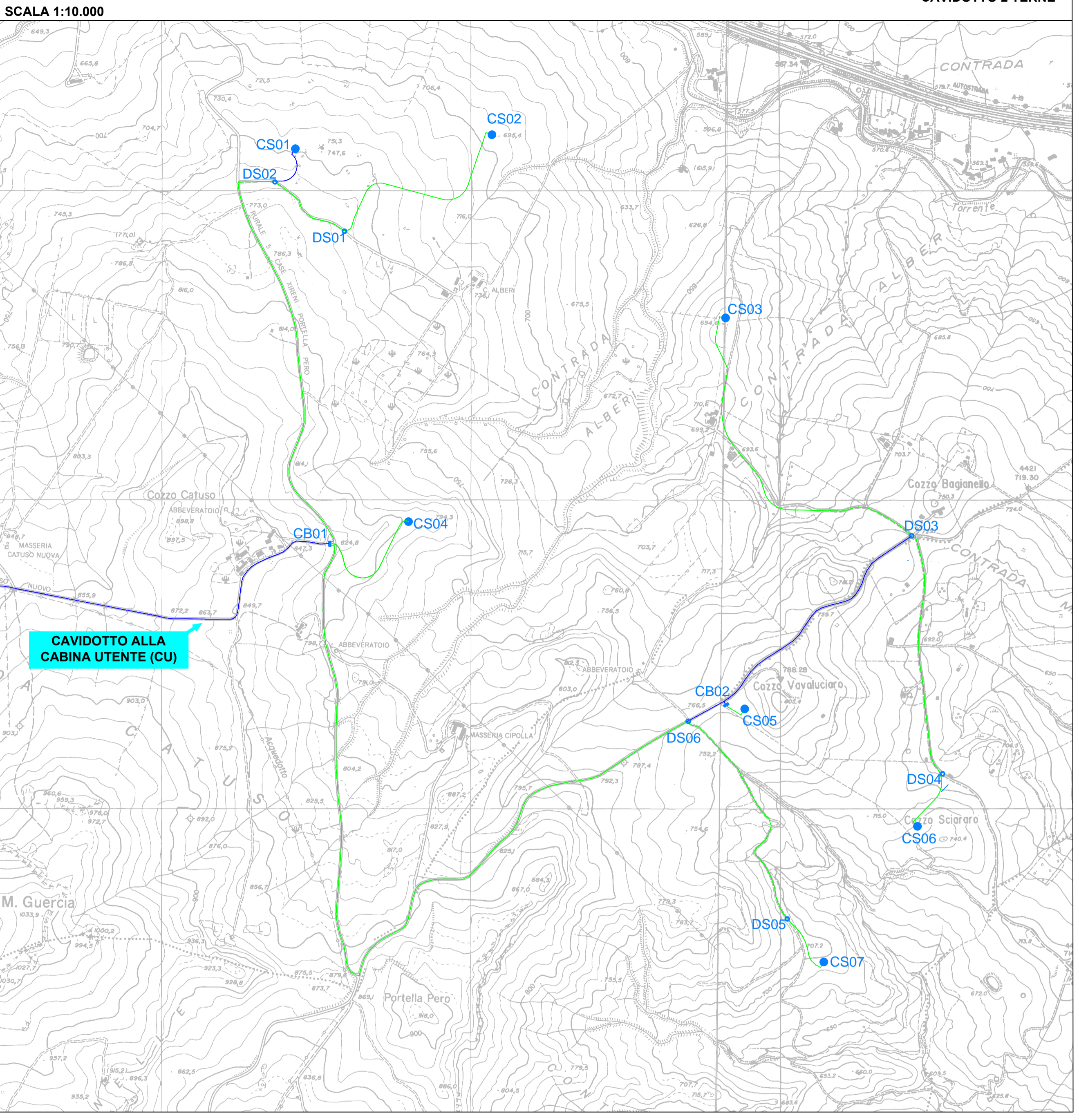
CAVIDOTTO 1 TERNA SU STRADA STERRATA
