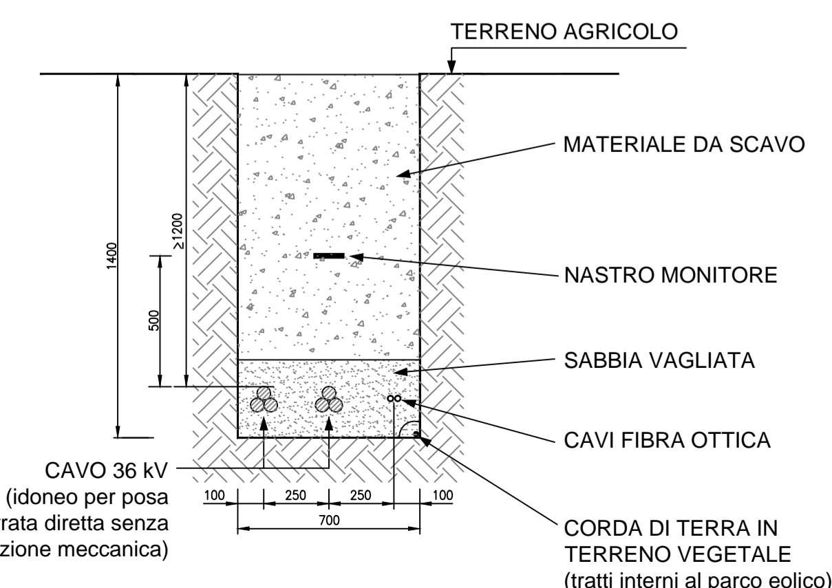
CAVIDOTTO 2 TERNA SU TERRENO AGRICOLO
