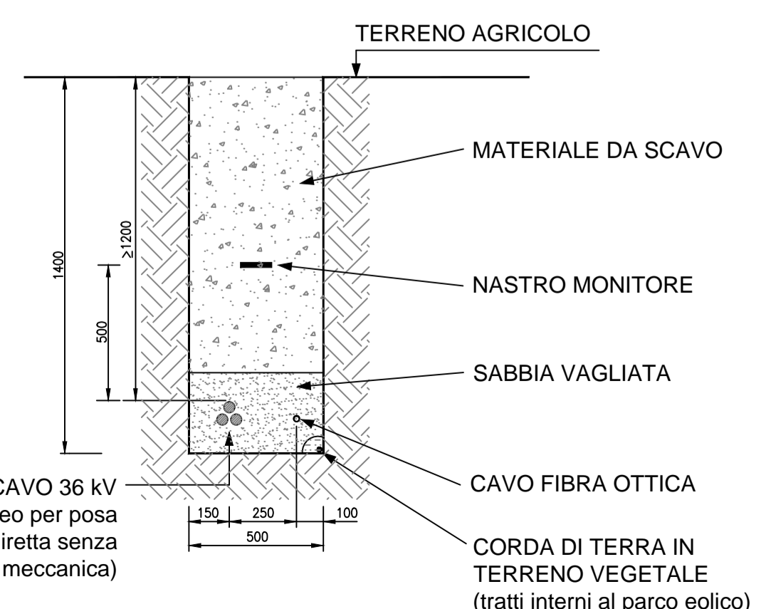
CAVIDOTTO 1 TERNA SU TERRENO AGRICOLO
