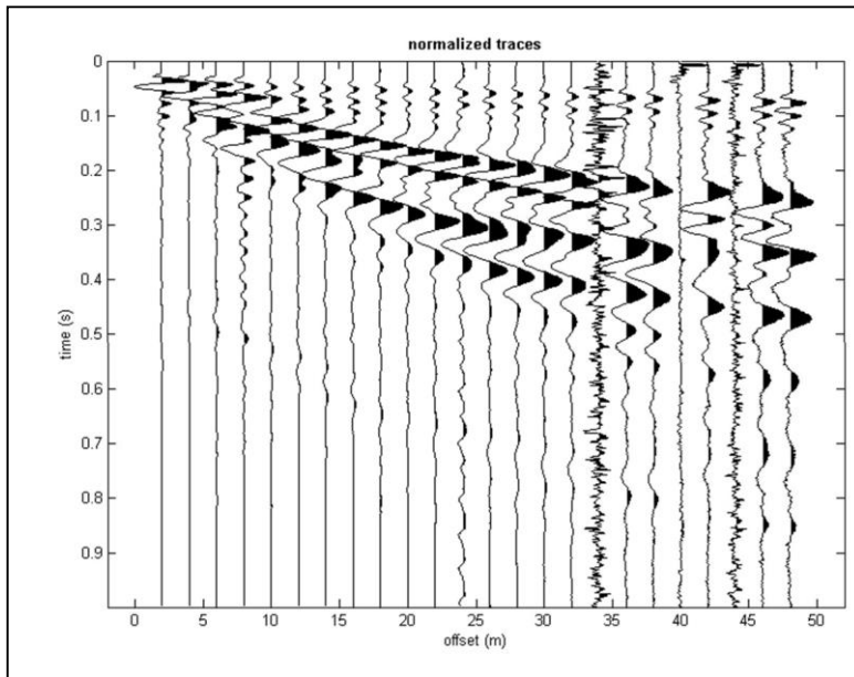
Figura 5: Tracce sperimentali
