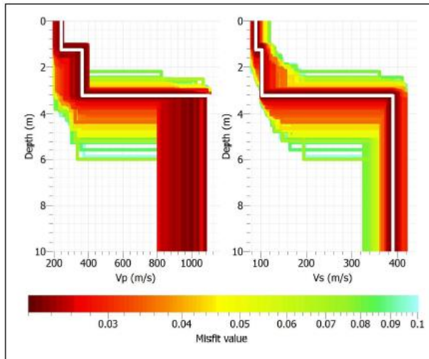
Figura 5: andamento delle Vp e delle Vs in funzione della profondità. In bianco il modello con la migliore attendibilità.
