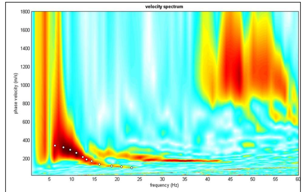
Figura 6: Spettro di velocità norm. e picking della curva di dispersione (punti bianchi)
