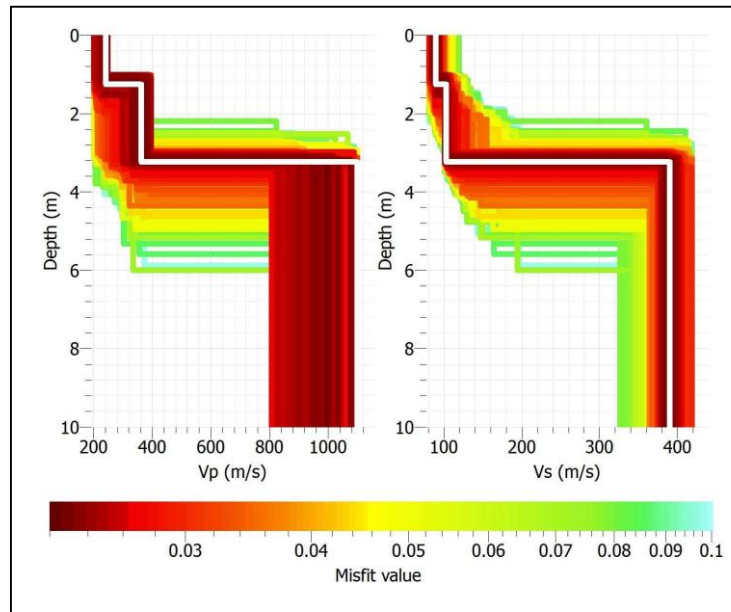
Figura 7: modelli 1D di velocità delle onde S e P (misfit max 10%), in bianco il modello con il miglior fit (best model)
