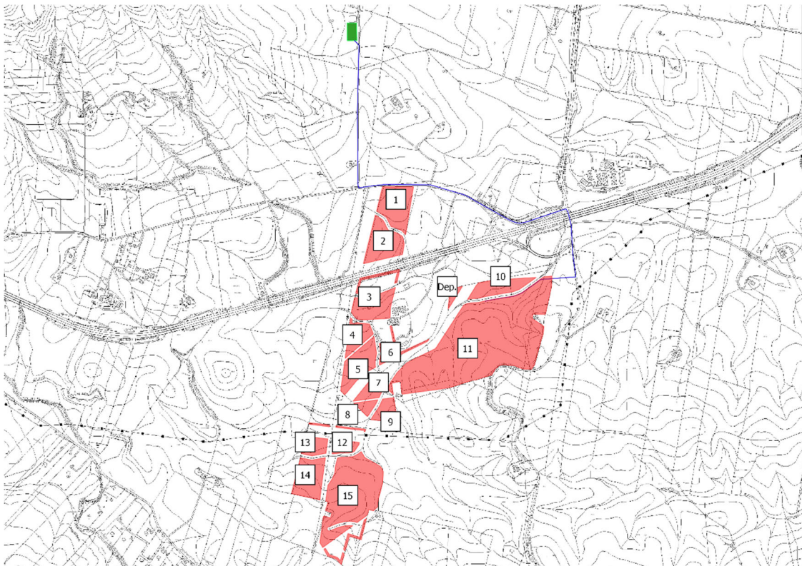
Figura 45 - Impianto agrivoltaico: indicazione dei sottocampi
