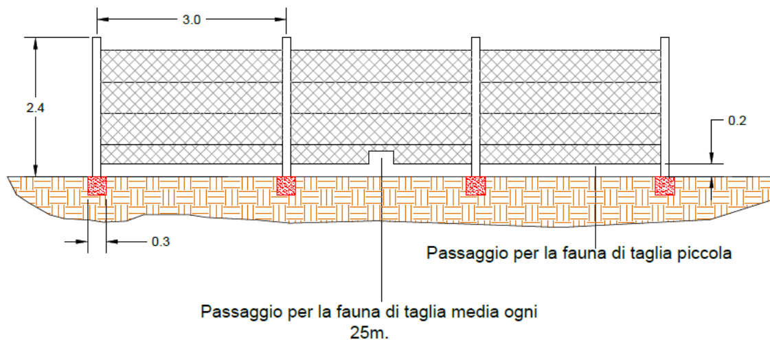
Figura 48 – Particolare della recinzione
