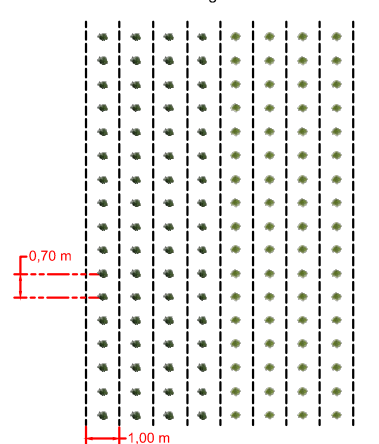
Posizionamento ala gocciolante nell'interfila
