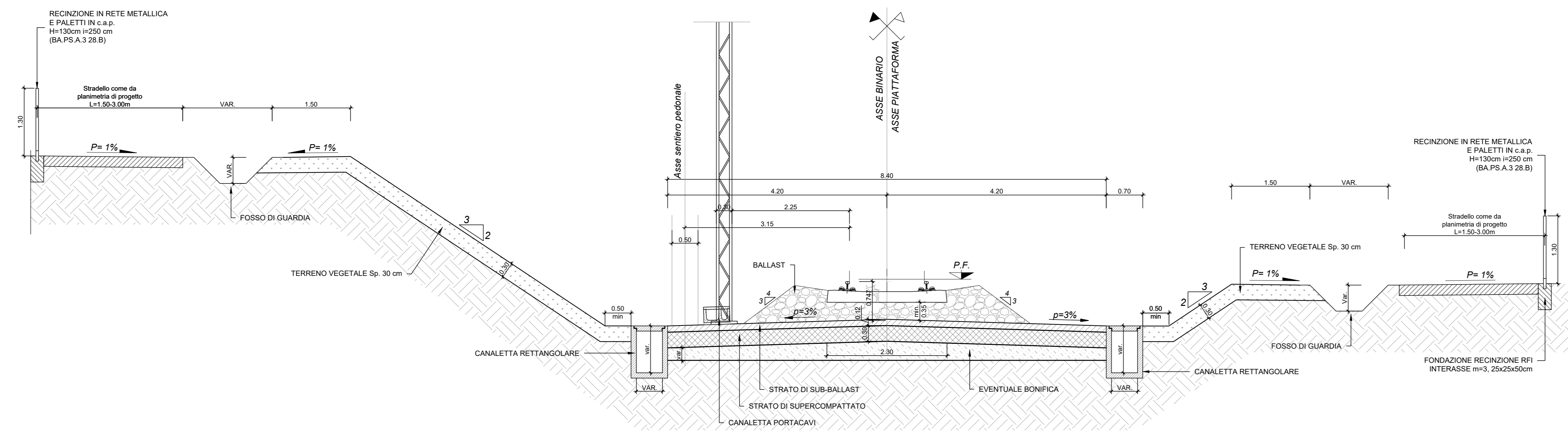
Sezione tipo a singolo binario in trincea - H_{tr} < 5,00 m SCALA 1:50
