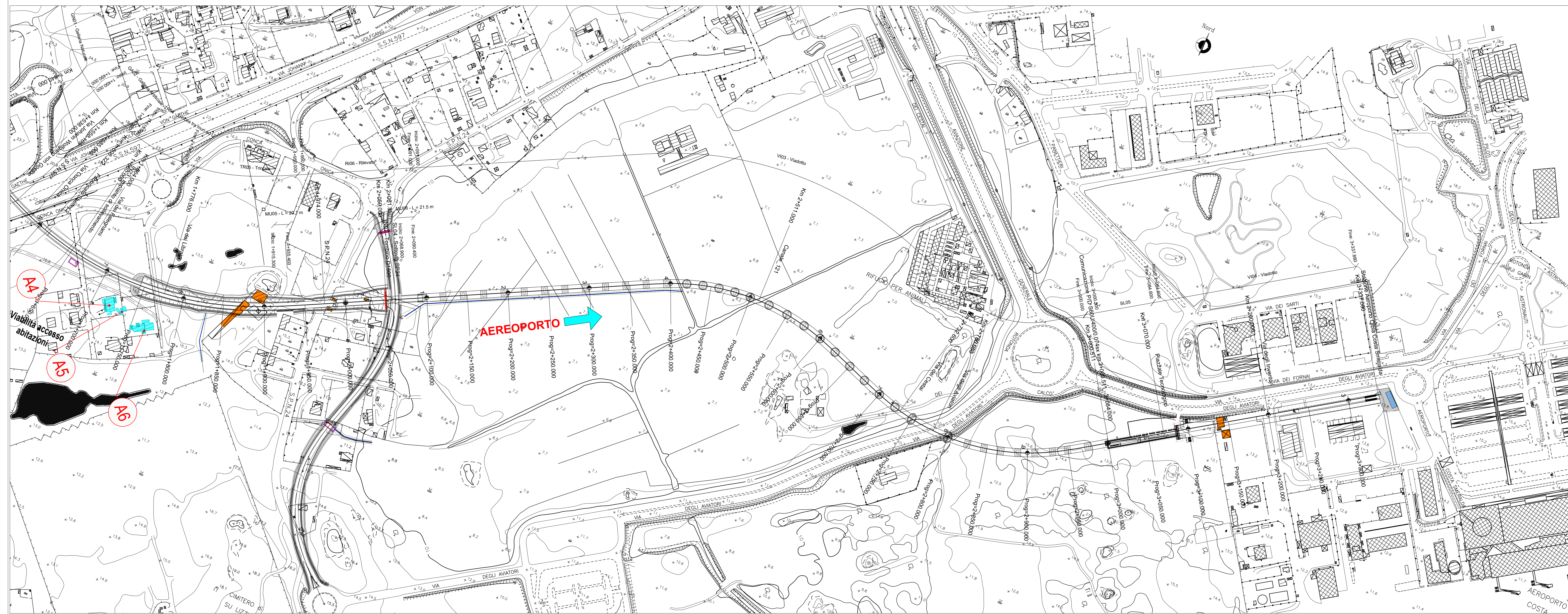
PLANIMETRIA DI PROGETTO 2/2 - Scala 1:2000
