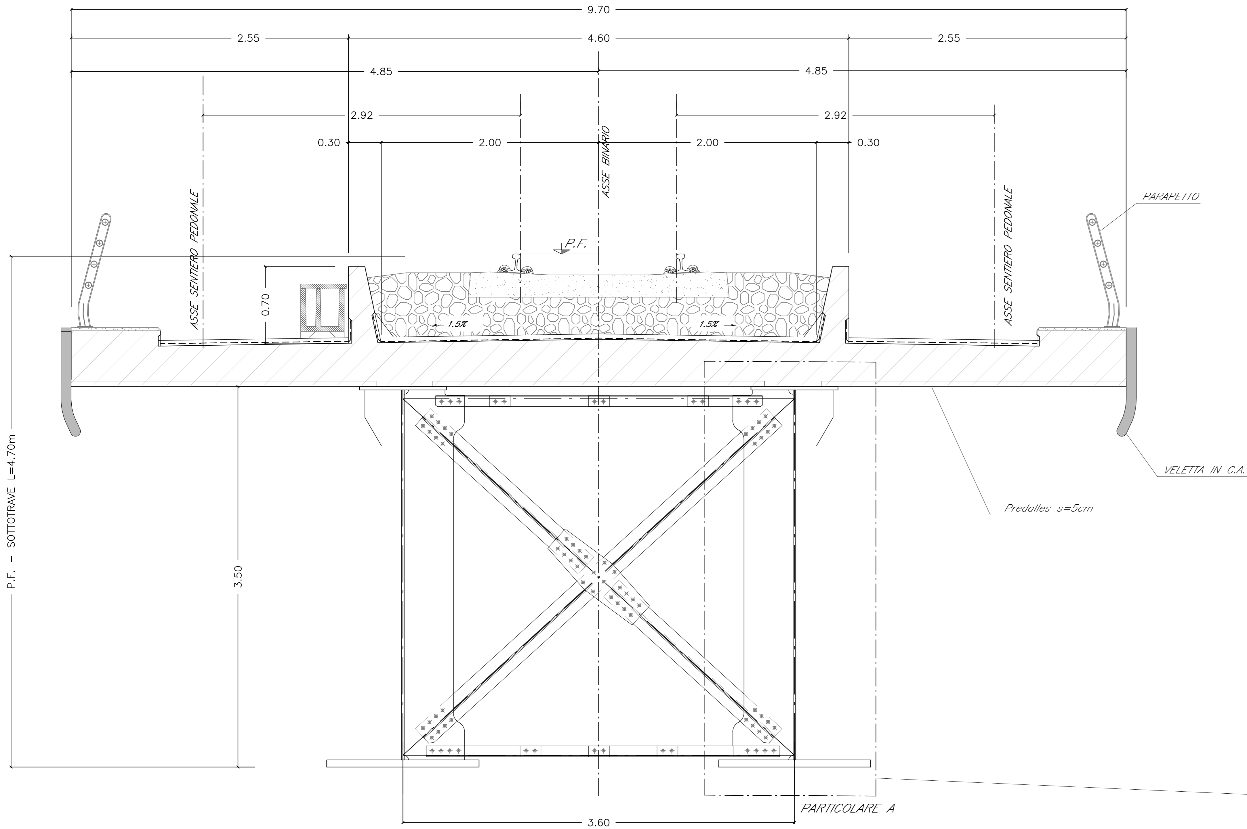
IMPALCATO. SEZIONE MISTA L=45m SINGOLO BINARIO SCALA 1:20
