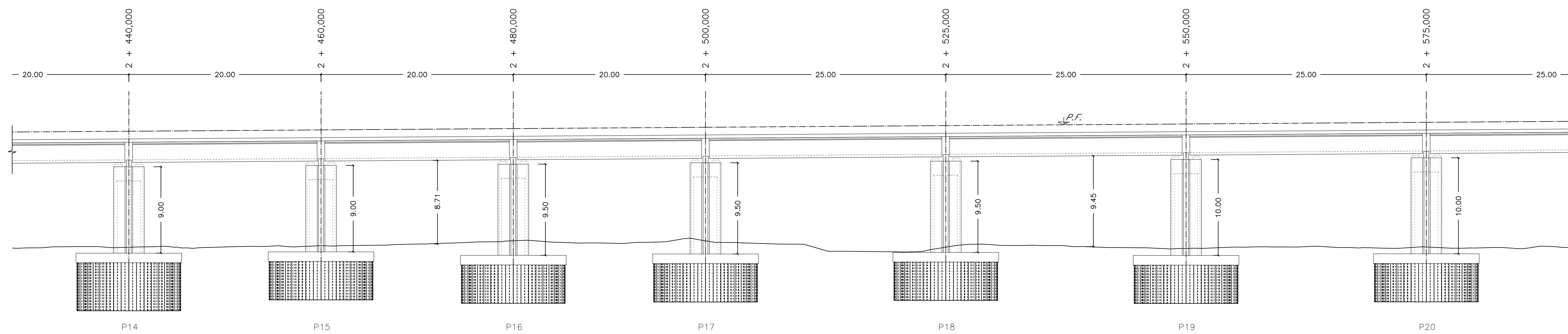
PROSPETTO VI03 SCALA 1:150
