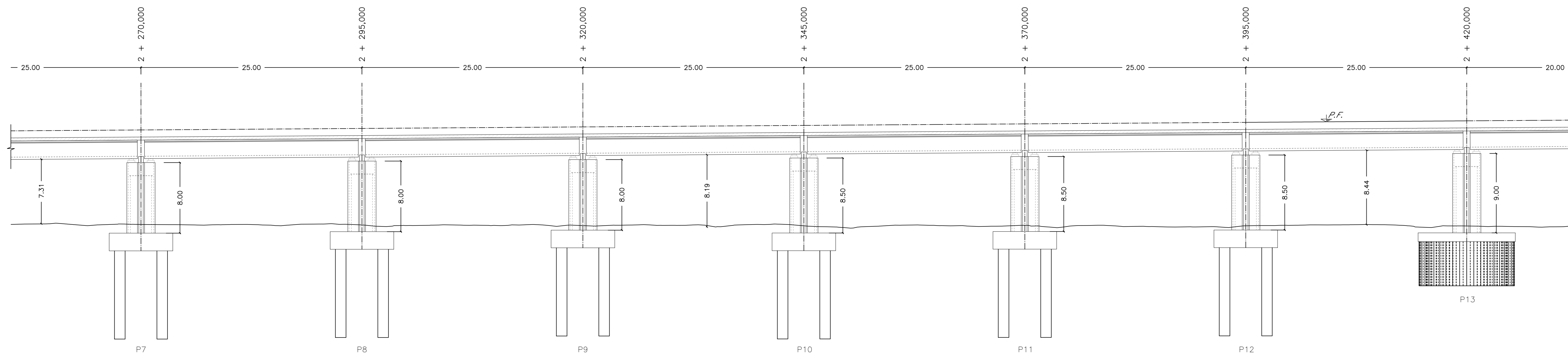
PROSPETTO VI03 SCALA 1:150
