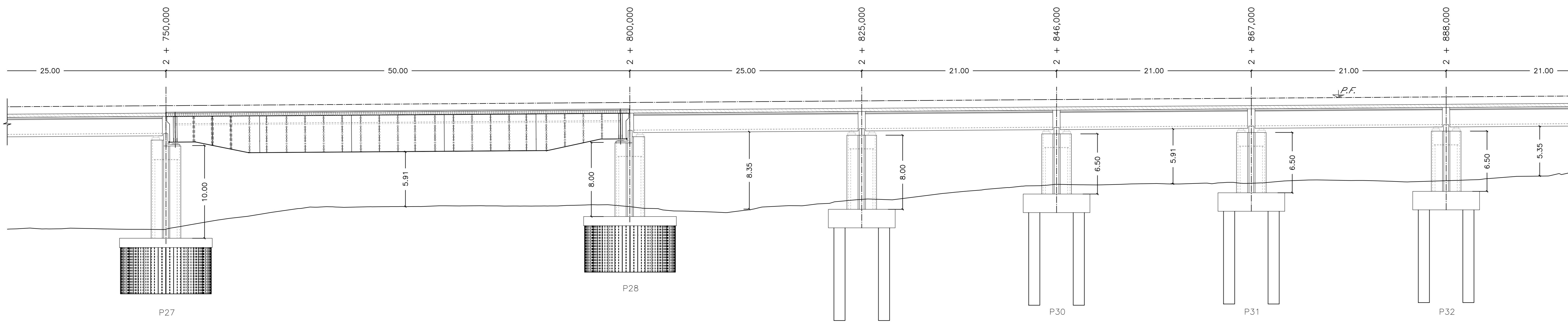
PROSPETTO VI03 SCALA 1:150
