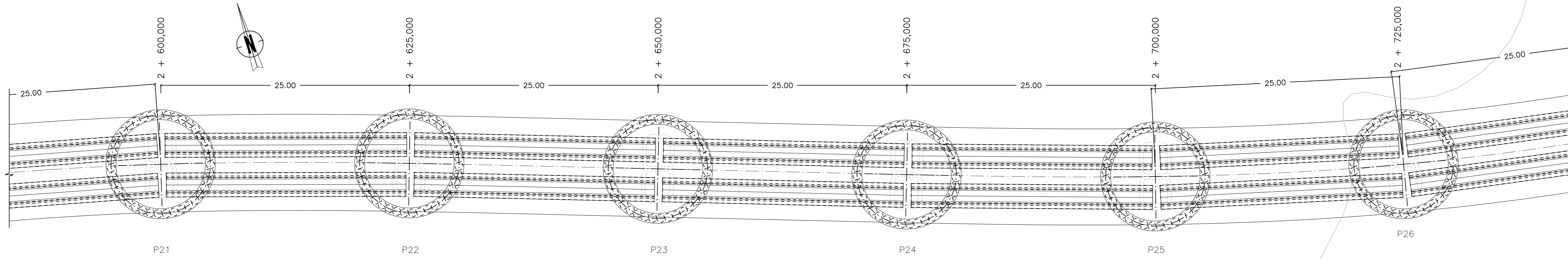
PIANTA VI03 SCALA 1:150
