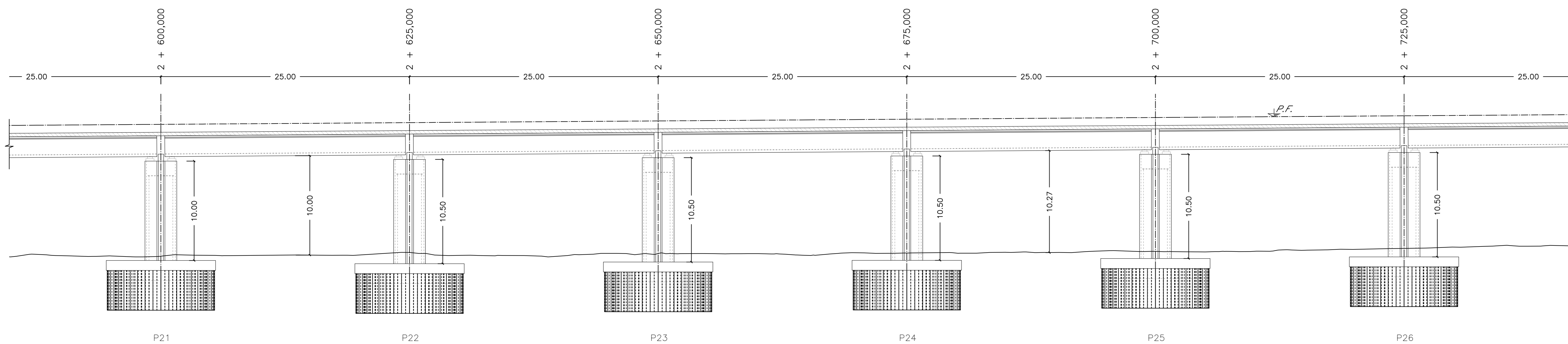
PROSPETTO VI03 SCALA 1:150
