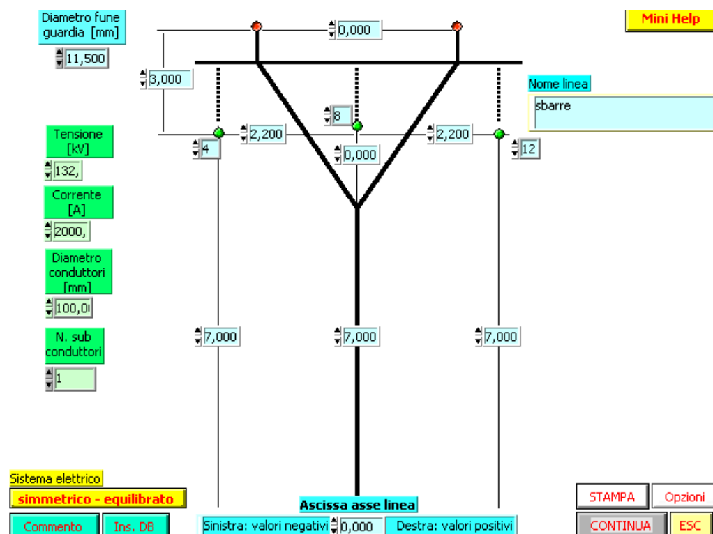
Figura 5: Linea AT con disposizione conduttori in piano assimilabile ad un sistema semplice sbarra a 132/150 kV
