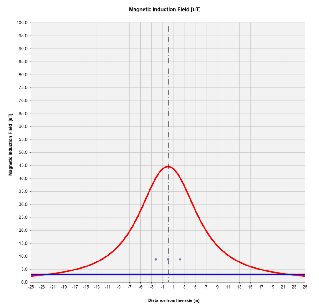
Figura 6: Andamento del campo di induzione magnetica per I = 2000 A
