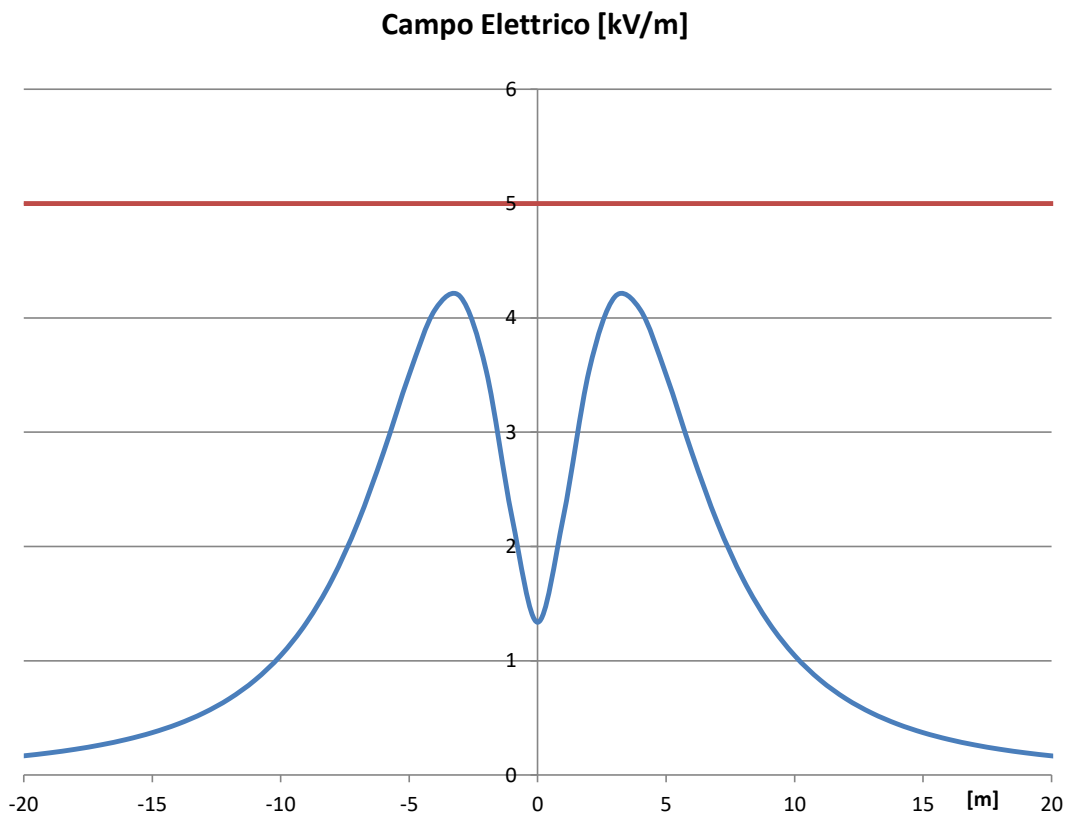
Figura 4: Campo elettrico al suolo generato dal sistema di sbarre a 150 kV
