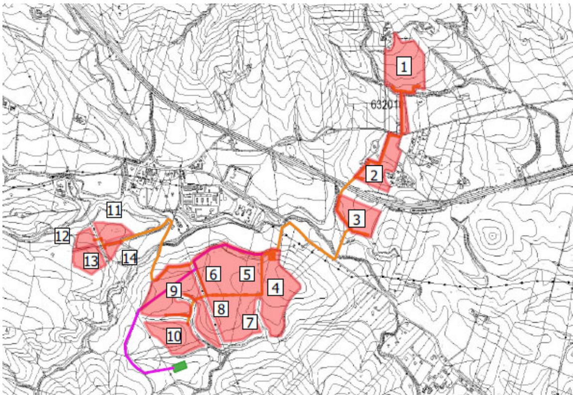
Figura 8 - Impianto agrivoltaico: indicazione dei sottocampi
