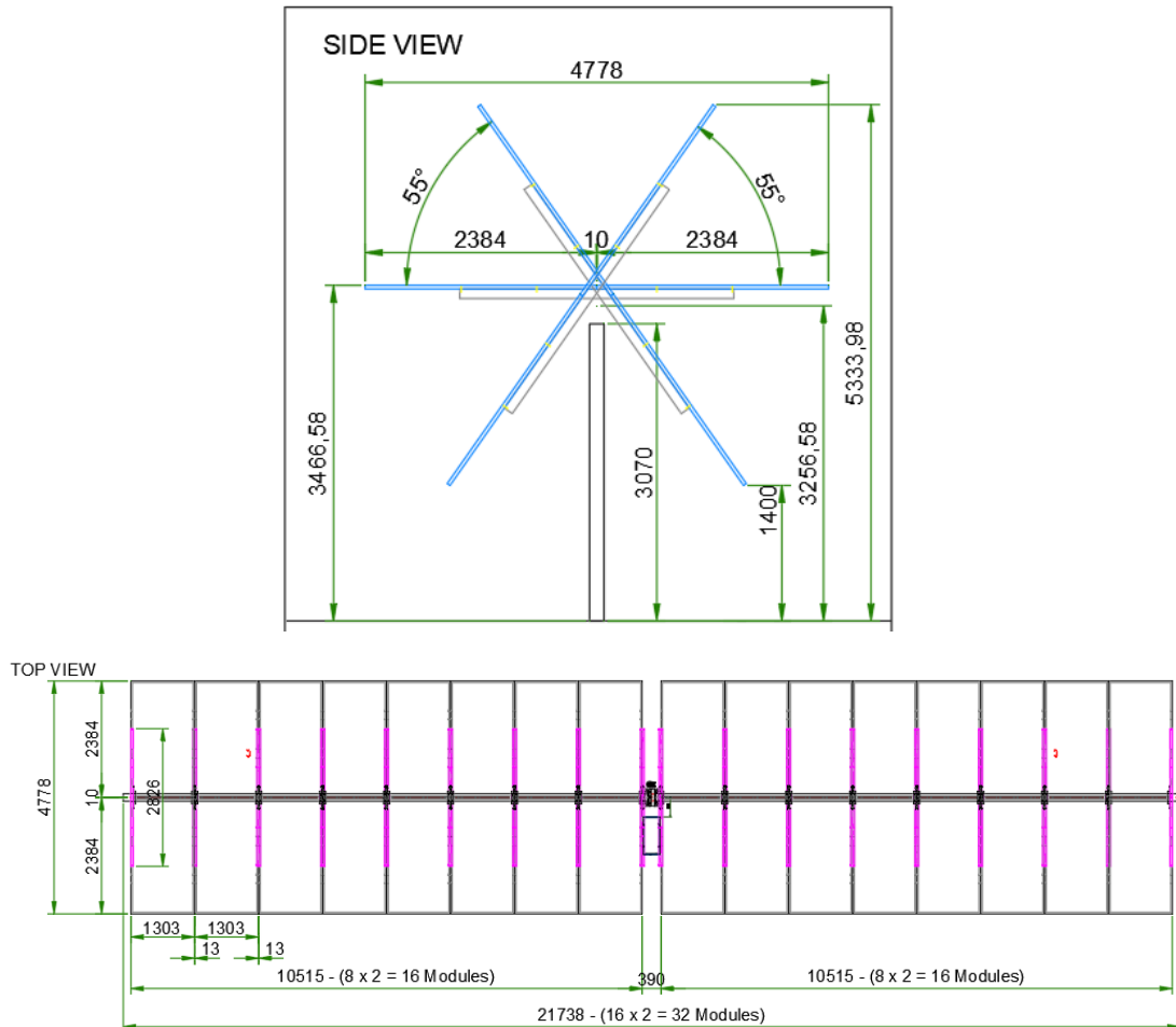
Figura 10 – Pannelli fotovoltaici
